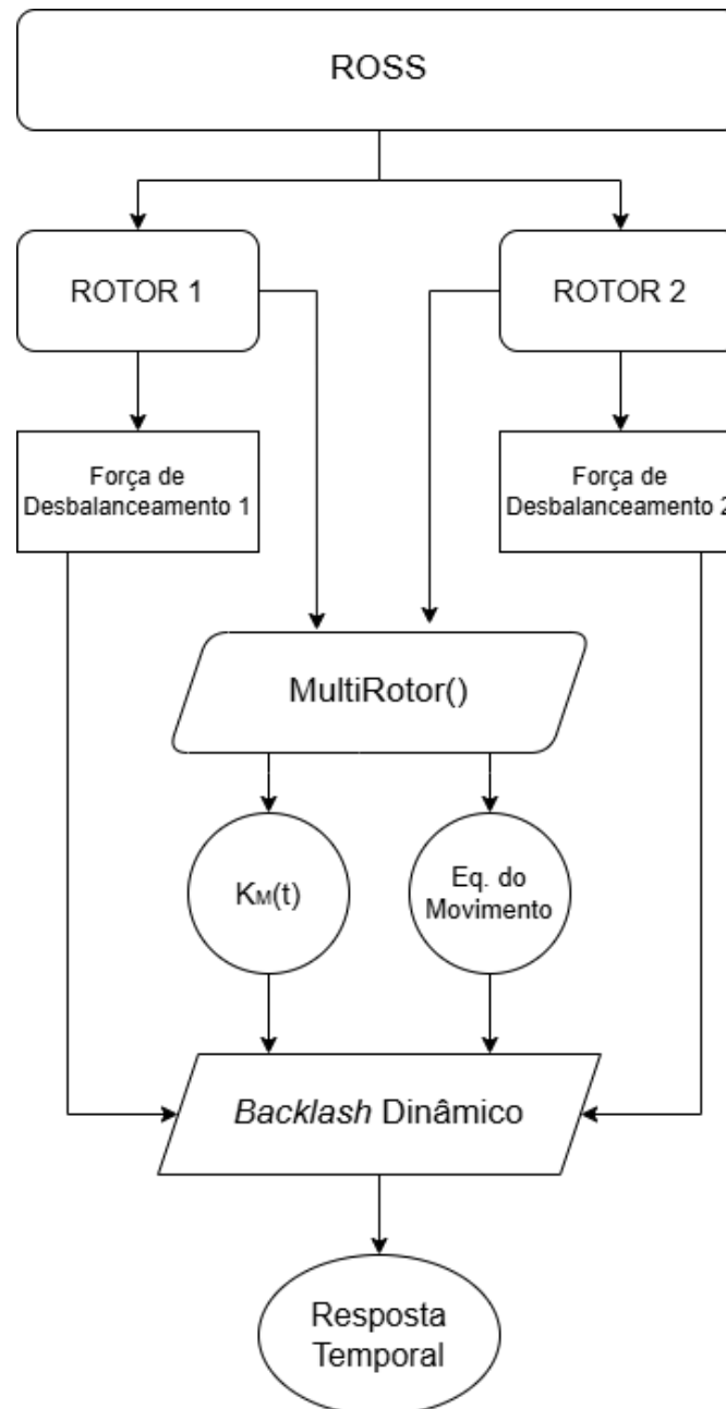
Figura 3.1 – Fluxograma de execução do código
