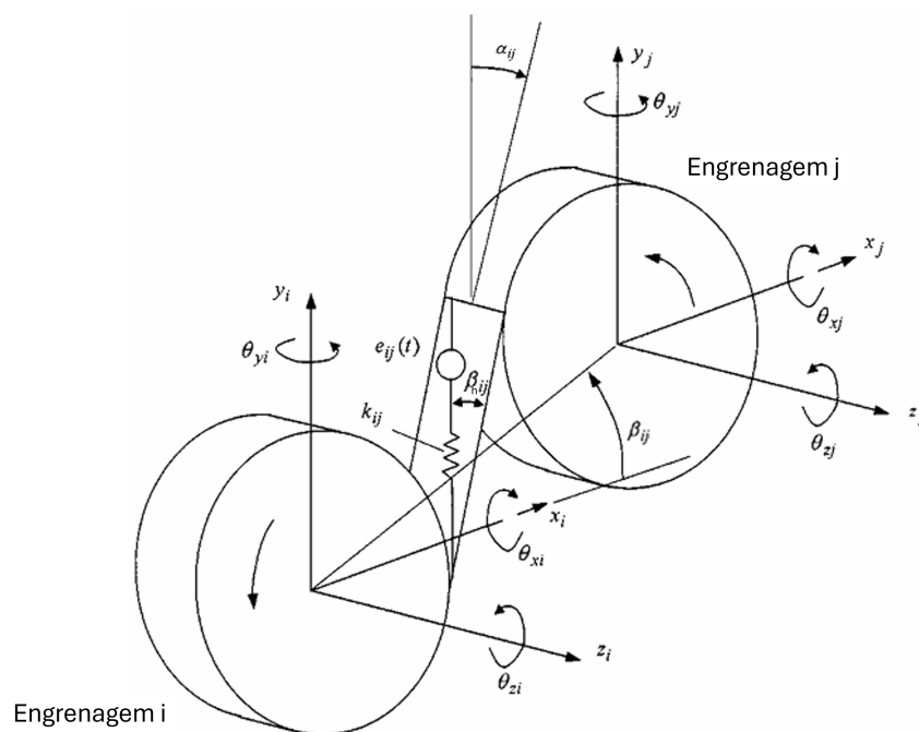
Figura 3.3 – Modelo de 6 gdl
