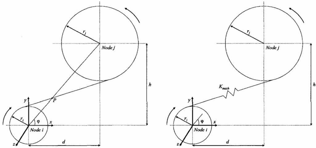
Figura 2.11 – Reapresentação do Engrenamento
