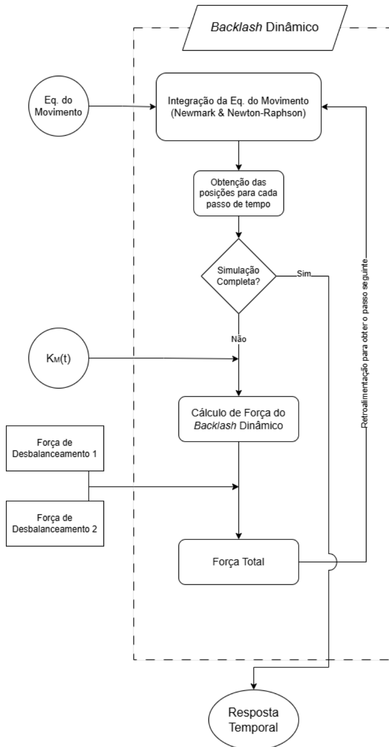
Figura 3.2 – Fluxograma interno de execução do código
