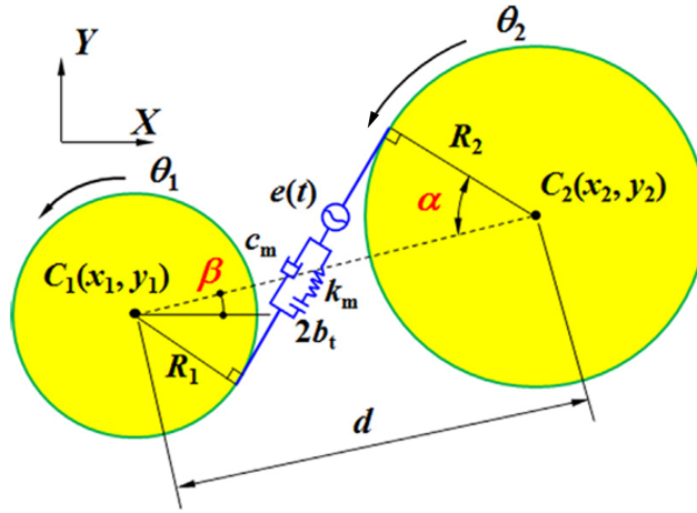
Figura 2.10 – Modelo de Par Engrenado
