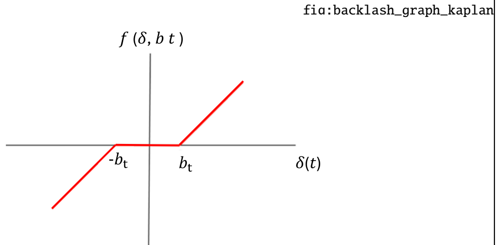
Figura 2.9 – Deformação da malha de engrenamento considerando a folga de backlash
