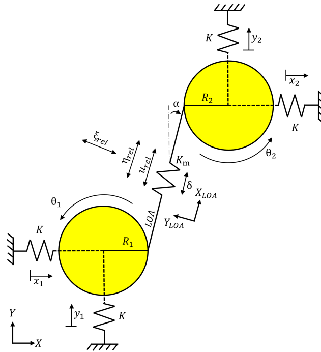
Figura 3.1 – Modelo analítico simplificado
