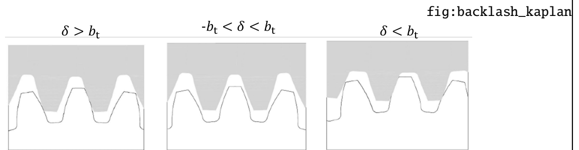
Figura 2.18 – Representação da folga de backlash
