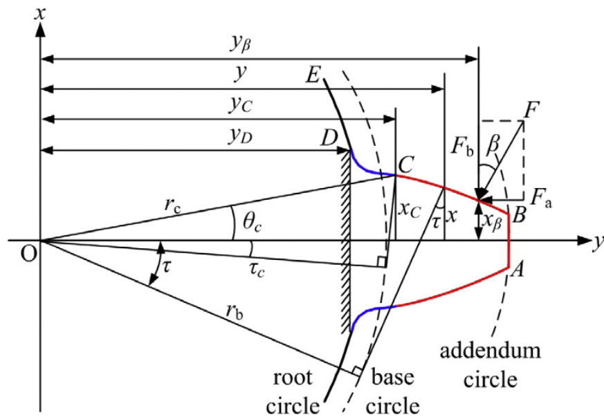
Figura 2.17 – Modelo geométrico do perfil do dente da engrenagem
