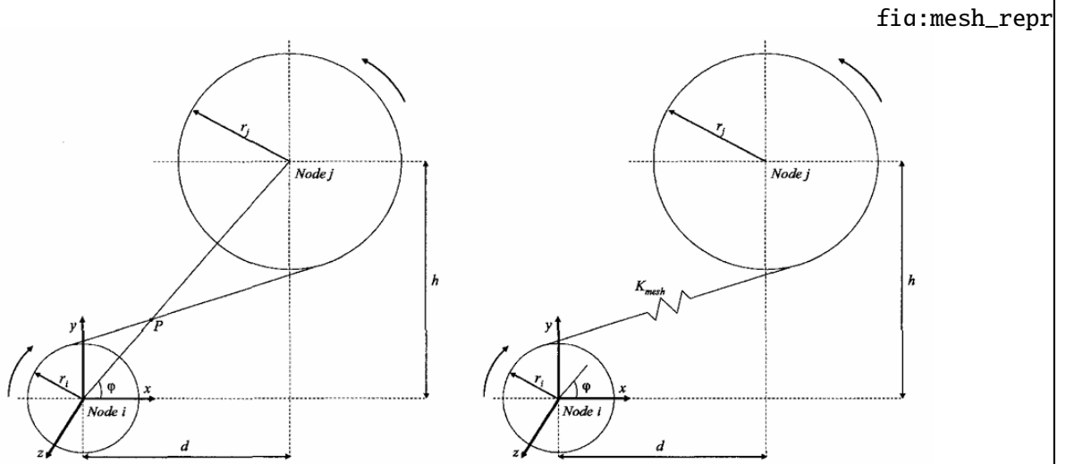
Figura 2.11 – Reapresentação do Engrenamento
