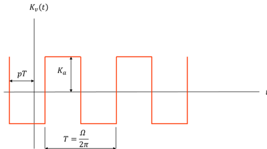
Figura 2.14 – Perfil de rigidez do engrenamento correlacionado com razão de contato
