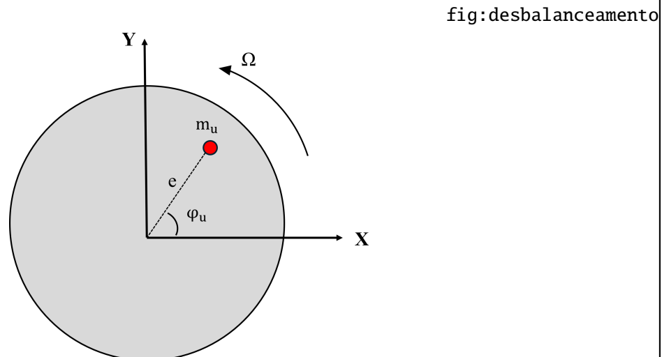
Figura 2.4 – Representação esquemática do desbalanceamento.
