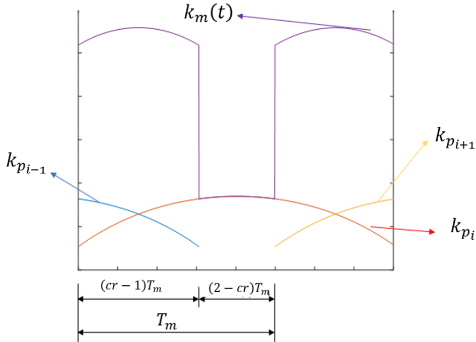
Figura 2.16 – Perfil de rigidez do engrenamento correlacionado com razão de contato
