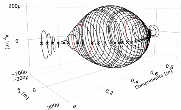
Figura 2.6 – Representação esquemática do desbalanceamento.
