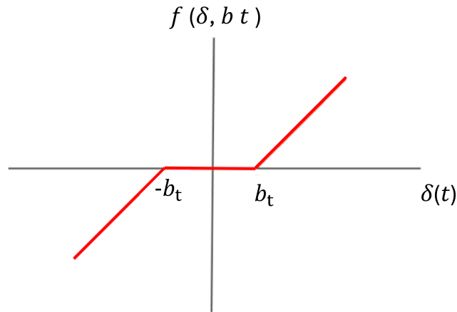
Figura 2.12 – Deformação da malha de engrenamento considerando a folga de backlash
