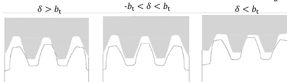
Figura 2.11 – Representação da folga de backlash
