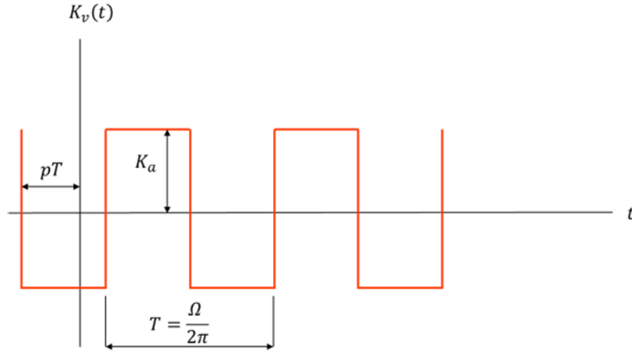
Figura 2.6 – Perfil de rigidez do engrenamento correlacionado com razao de contato
