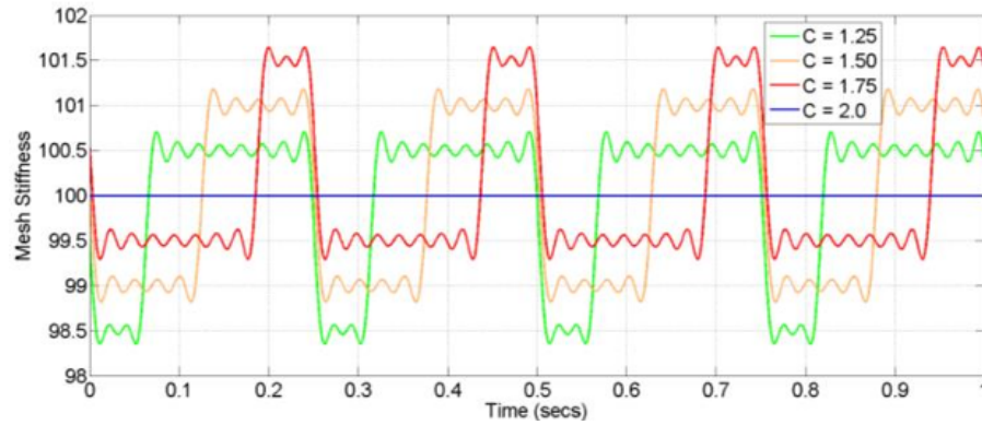
Figura 2.7 – Perfil de rigidez do engrenamento correlacionado com razao de contato
