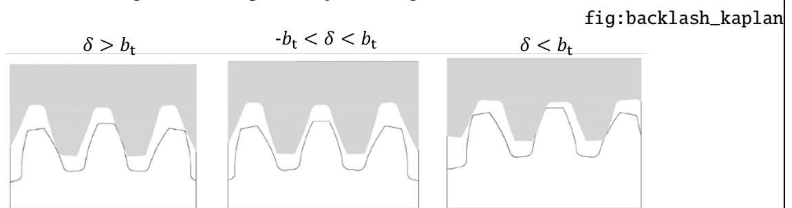
Figura 2.8 – Representação da folga de backlash
