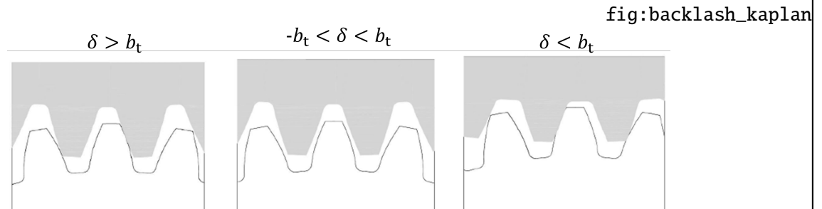
Figura 2.10 – Representação da folga de backlash
