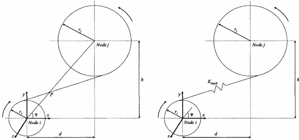
Figura 2.3 – Reapresentação do Engrenamento (KAPLAN, 2012)
