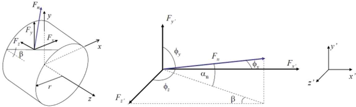
Figura 2.5 – Decomposição das forças no ponto de contato das engrenagens.
