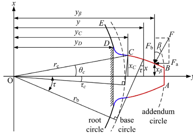
Figura 2.9 – Modelo geométrico do perfil do dente da engrenagem
