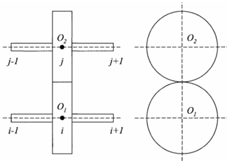
Figura 2.4 – Representação do par engrenado em elementos finitos (STRINGER, 2008)
