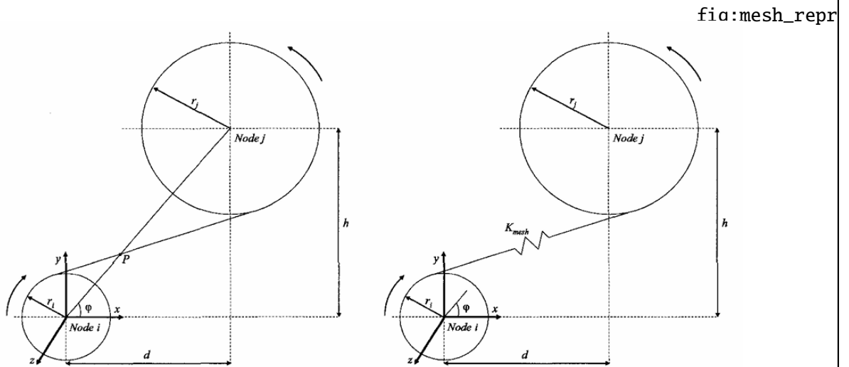
Figura 2.4 – Reapresentação do Engrenamento
