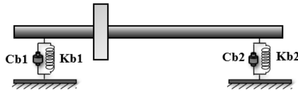
(a) Esquema de rotor
