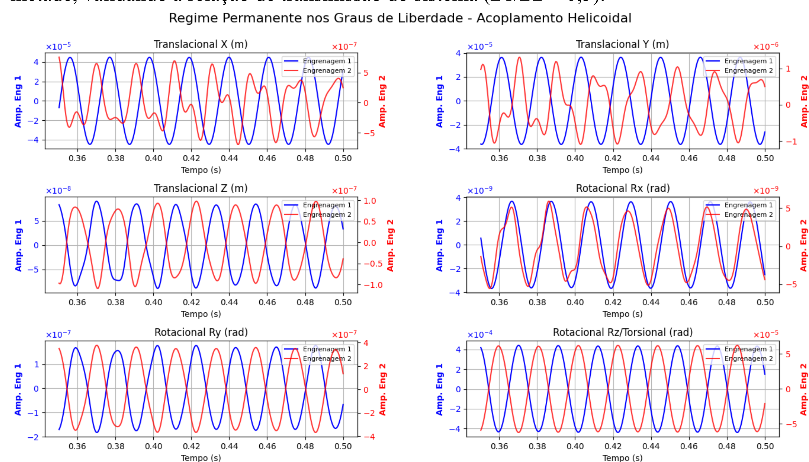
Figura 1: Resposta vibratória nos seis graus de liberdade para as engrenagens acopladas.
