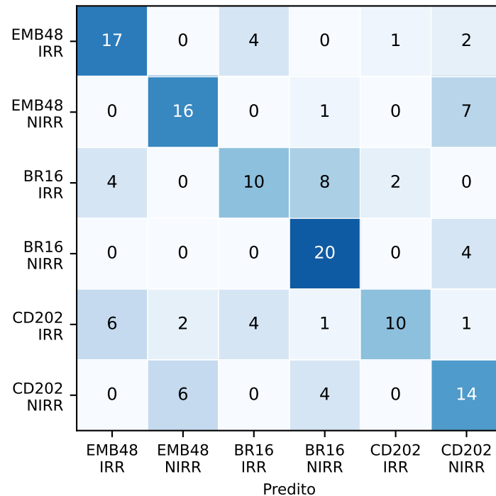
07_subset_bandas
