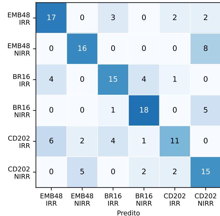
08_optuna_subset
