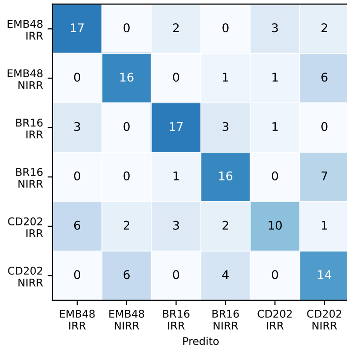
04_classificacao
