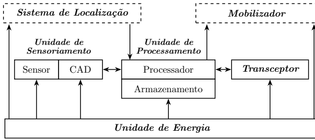
Figura 3. Componentes de um nó sensor. Adaptado de [4].
