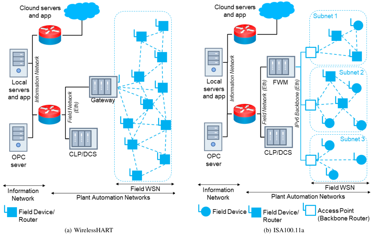
Figura 2. Arquiteturas de rede para aplicação em Indústria 4.0. Retirado de [3].
