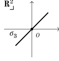
図3 \sigma_3 の接空間
