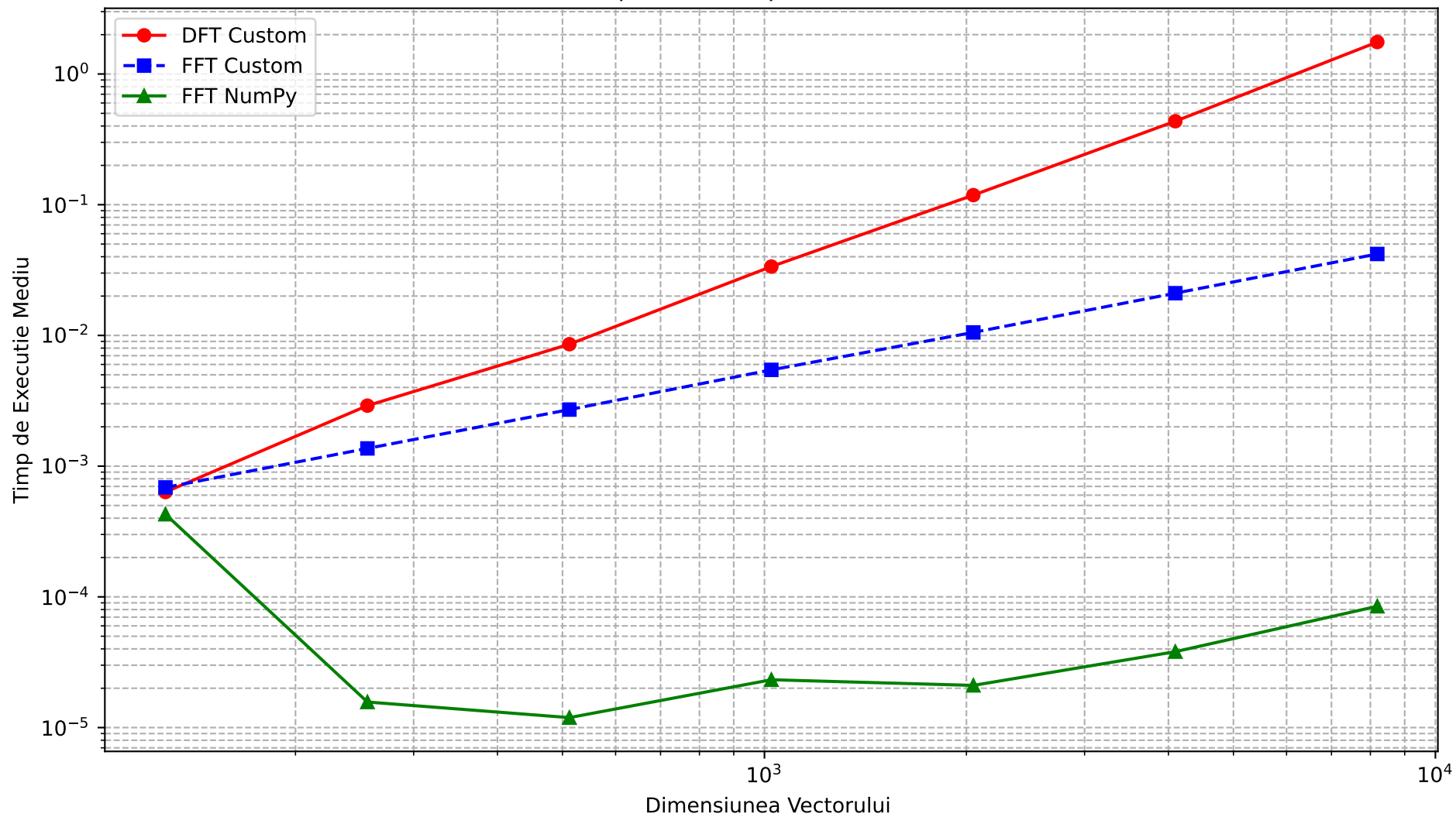
Compararea Timpului de Executie
