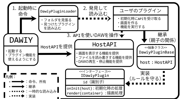
図 5: プラグイン周辺のクラス構造と連携
