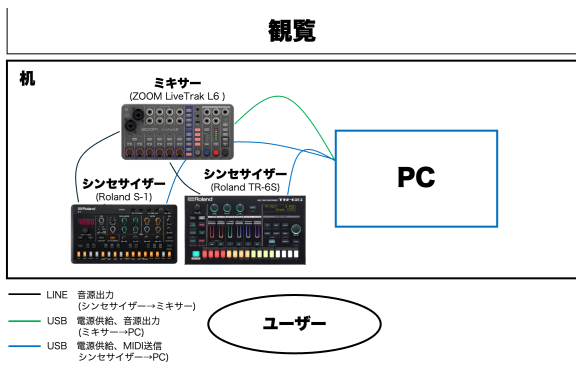
図 18: 使用機材の配置
