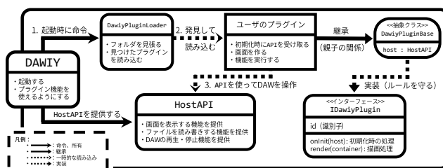
図 5: プラグイン周辺のクラス構造と連携
