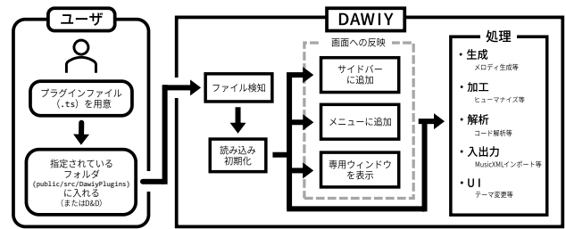
図 3: DAWIY プラグイン導入の流れ
