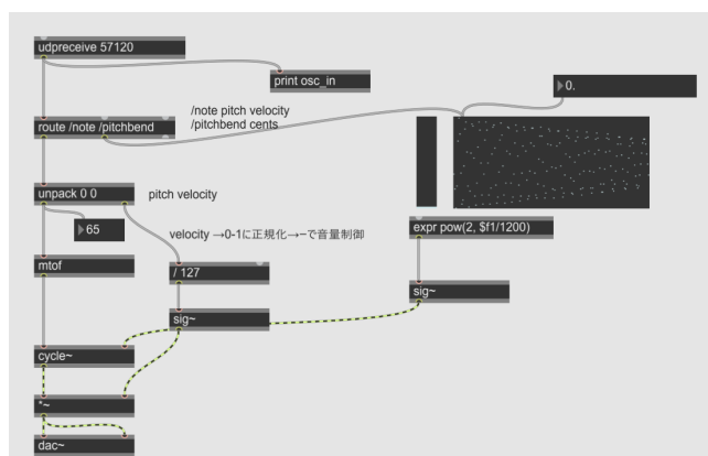
図 5: Max 8 構成
