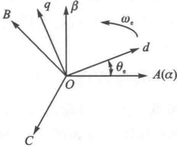
图 1-1: 三种坐标关系图
