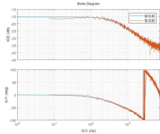
图 4-33: D 轴工作点-2V 数值解和解析解对比
