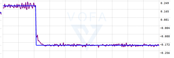
图 3-13: I_d=-0.2A 阶跃响应图
