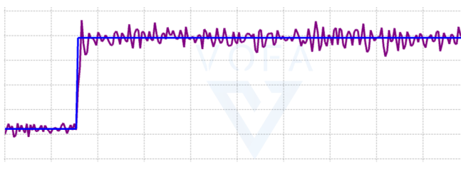
图 3-12: I_d=0.2A 阶跃响应图
