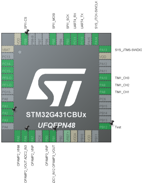
图 3-8: 外设配置图
