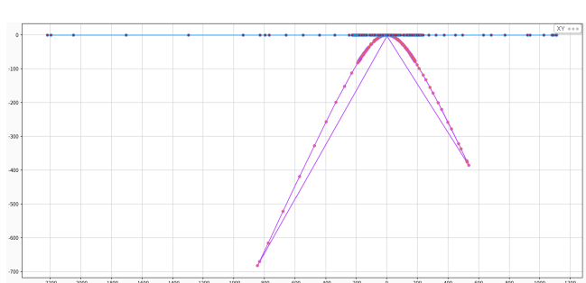
图 6-7: MTPA 仿真给定电流轨迹波形
