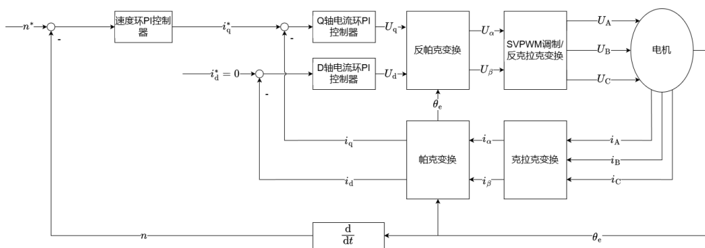
图 3-1: 经典 FOC 控制结构框图
