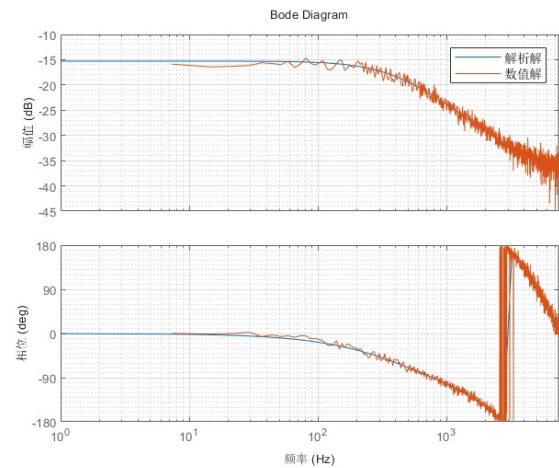
图 4-35: D 轴工作点-4V 数值解和解析解对比
