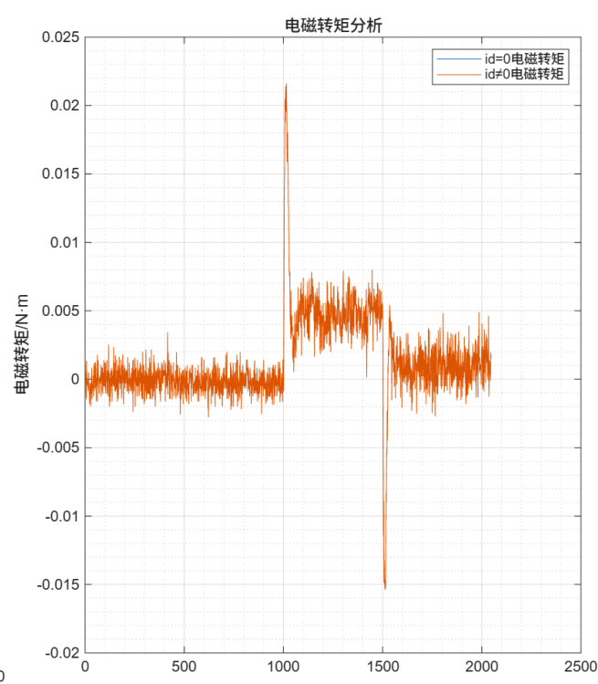
图 5-42: 速度环正向闭环方波电磁转矩对比
