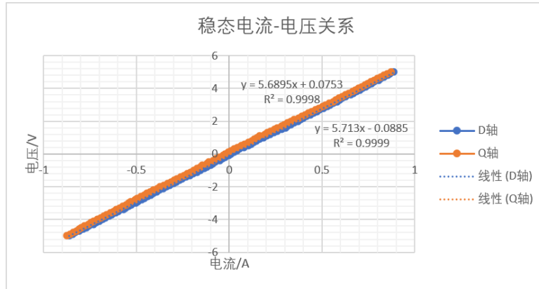
图 4-1: 相电阻辨识曲线
