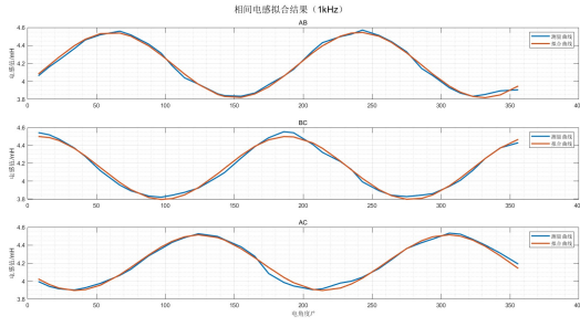
图 4-4: 1kHz 相间电感拟合结果
