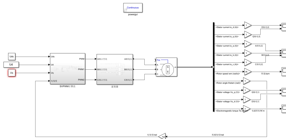
图 4-6: 仿真模型
