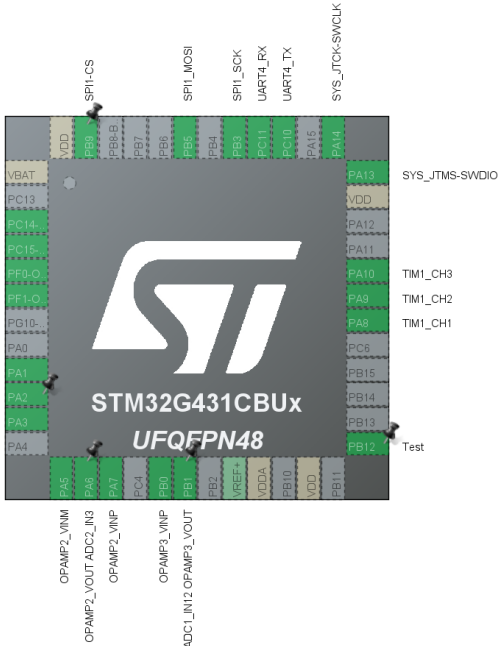
图 3-8: 外设配置图
