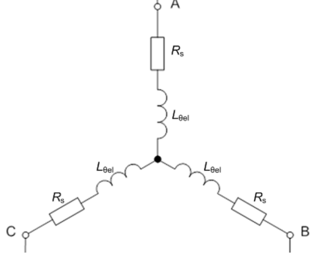
图 1-2: 三相电机电路图
