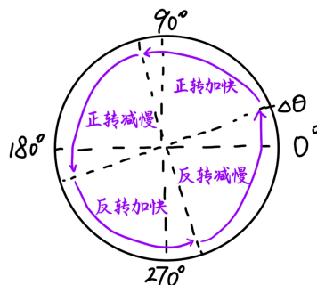
图 3-10: 粗校准过程
