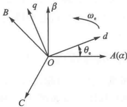
图 1-4: 帕克变换
