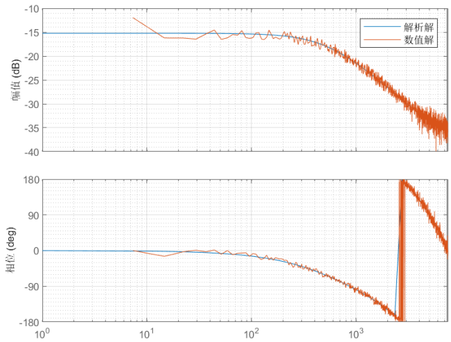
图 4-31: D 轴工作点 4V 数值解和解析解对比
