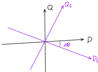
图 3-9: 控制坐标系和实际坐标系
