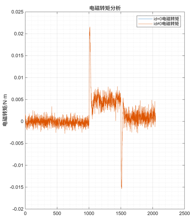
图 5-42: 速度环正向闭环方波电磁转矩对比
