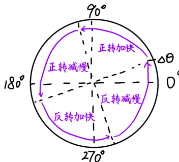
图 3-10: 粗校准过程
