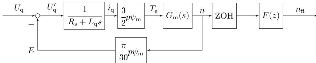
图 5-28: i_d = 0 假设下的 Q 轴电流-速度系统框图（带低通滤波器）
