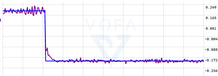
图 3-13: I_d=-0.2A 阶跃响应图
