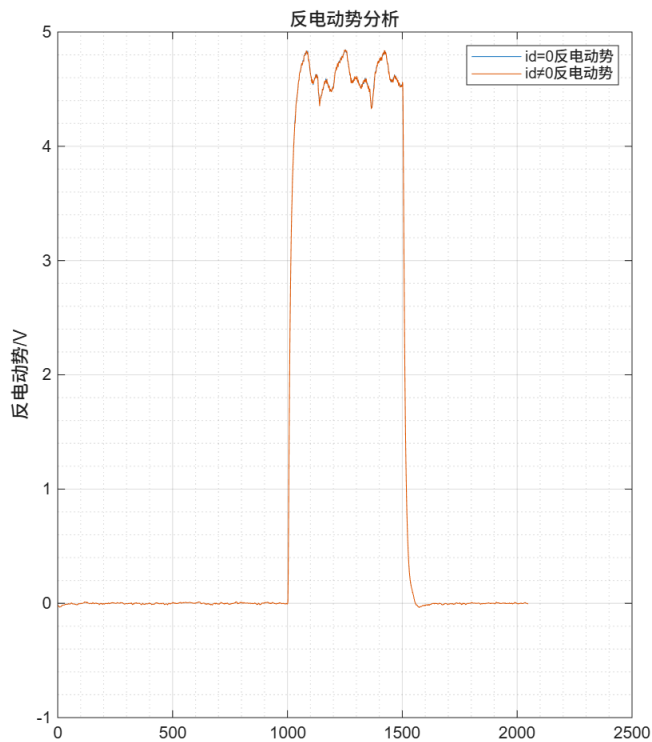
图 5-29: 速度环正向方波反电动势对比
