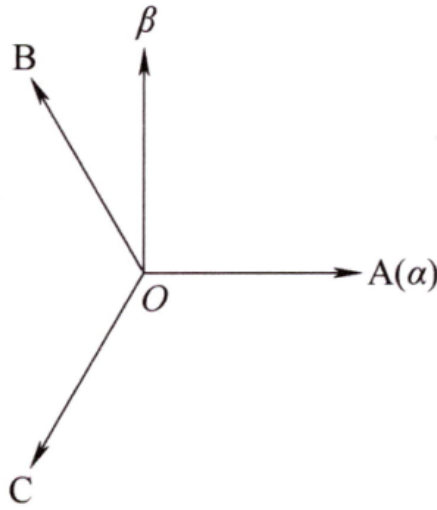
图 1-3: 克拉克变换
