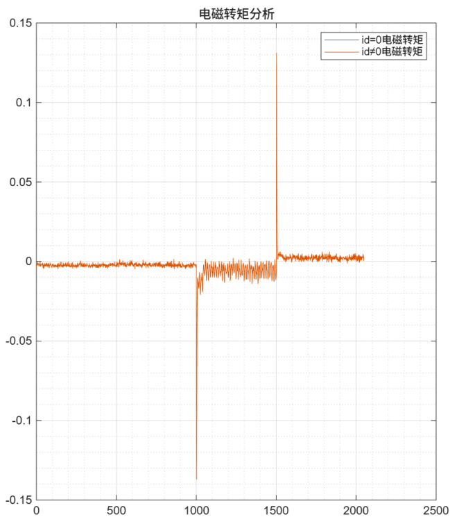
图 5-33: 速度环负向方波电磁转矩对比
