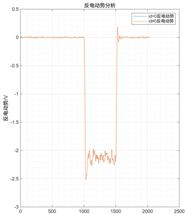
图 5-43: 速度环负向闭环方波反电动势对比
