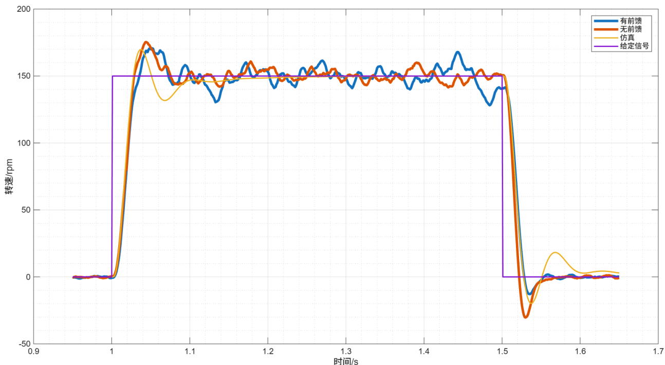
图 5-46: 前馈补偿对比
