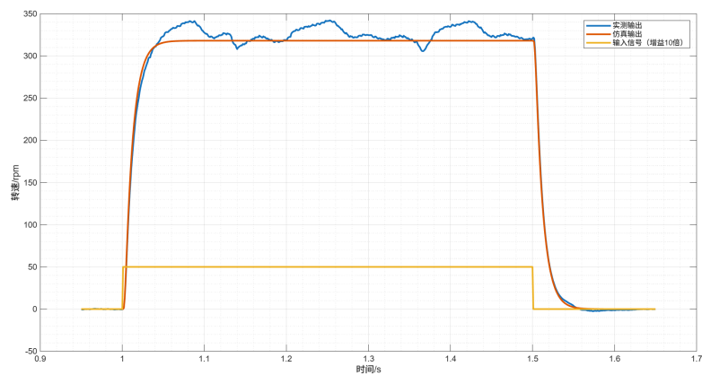
图 5-31: 速度环正向方波转速对比
