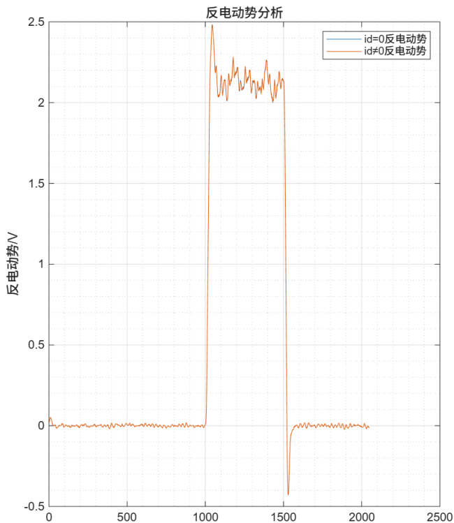
图 5-41: 速度环正向闭环方波反电动势对比
