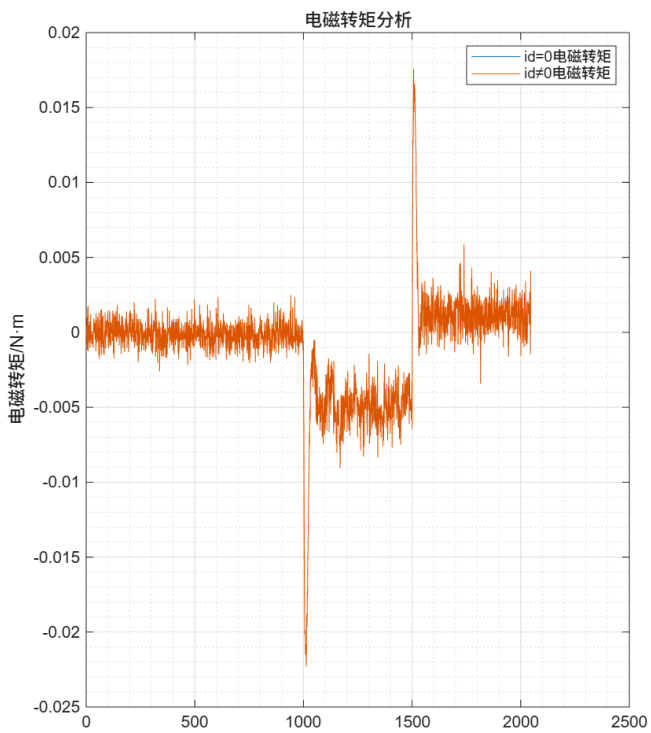
图 5-44: 速度环负向闭环方波电磁转矩对比
