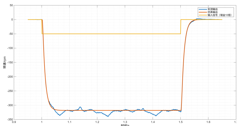
图 5-34: 速度环负向方波转速对比
