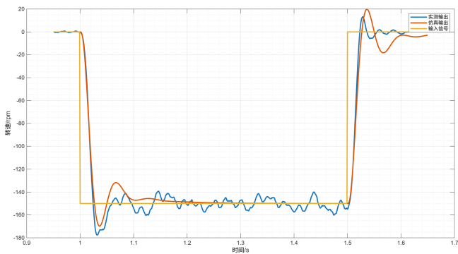
图 5-40: 速度环负向方波闭环验证
