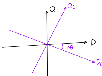
图 3-9: 控制坐标系和实际坐标系
