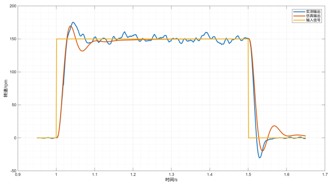
图 5-39: 速度环正向方波闭环验证
