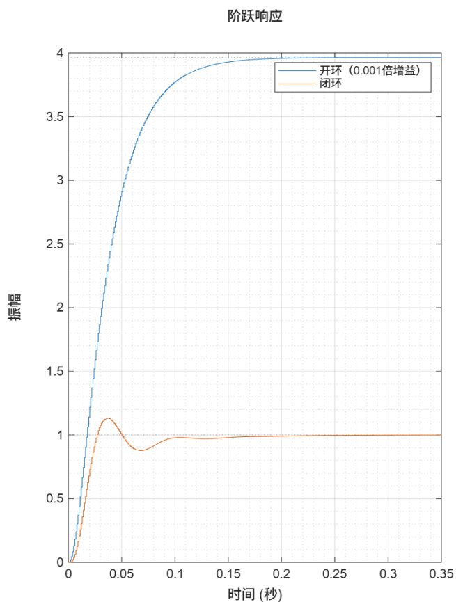
图 5-38: 速度环开-闭环单位阶跃响应对比
