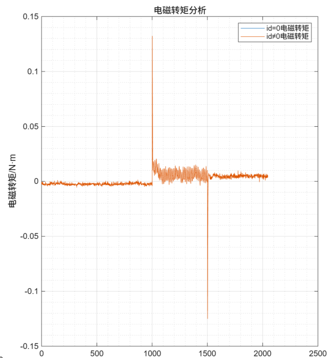
图 5-30: 速度环正向方波电磁转矩对比
