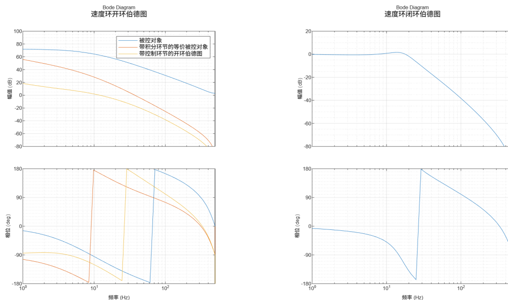
图 5-37: 速度环开-闭环频率特性
