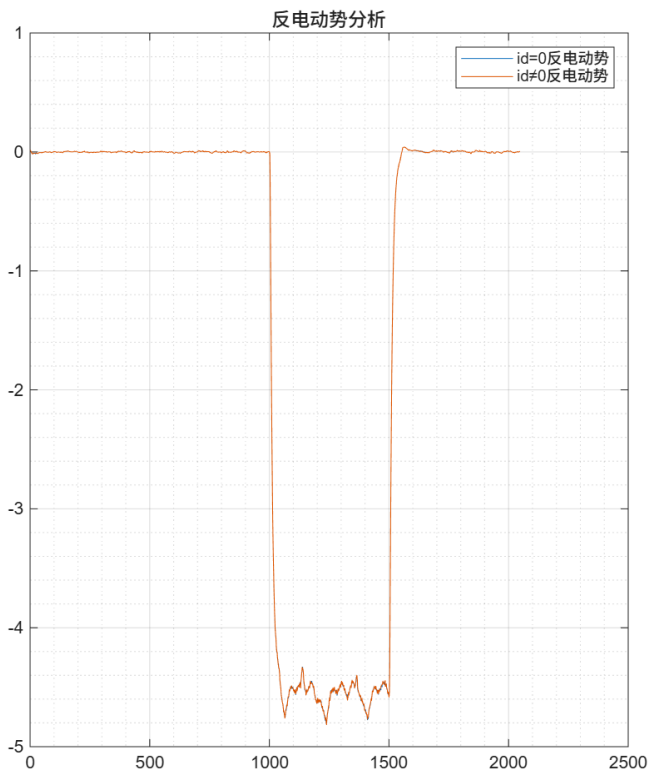
图 5-32: 速度环负向方波反电动势对比
