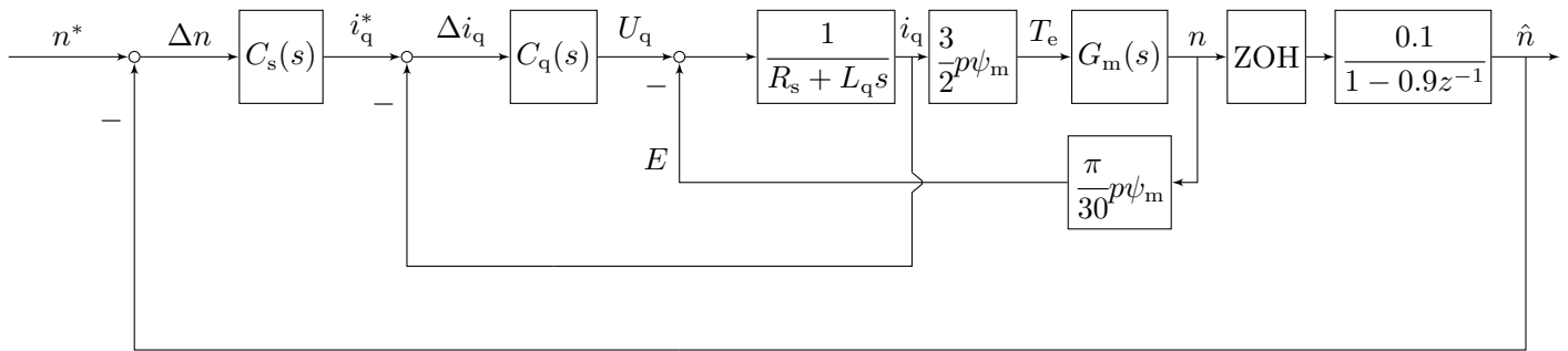
图 5-35: Q 轴双闭环控制系统框图
