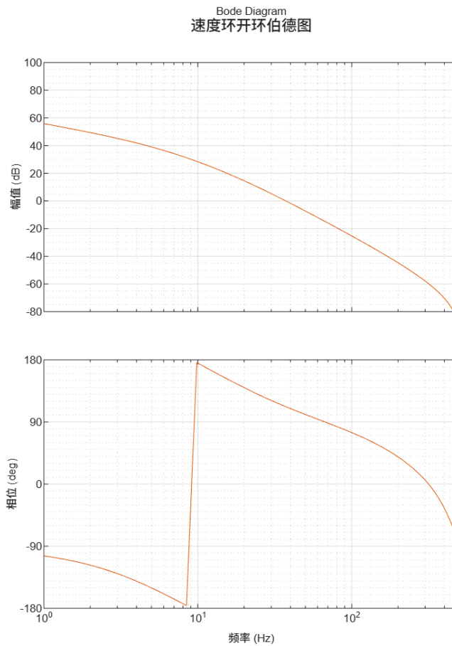
图 5-36: 带积分环节的速度环等价被控对象开环频率特性
