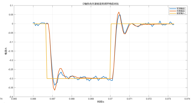
图 5-5: D 轴负向方波闭环验证
