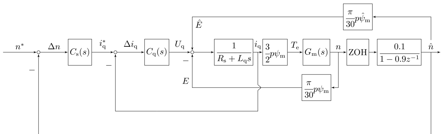
图 5-45: Q 轴双闭环控制系统框图
