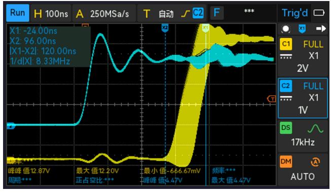
图 4-9: DRV8313 逆变器输出时序波形（惯性）
