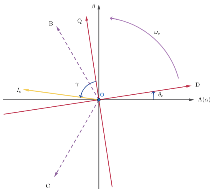
图 6-1: 电流超前角定义
