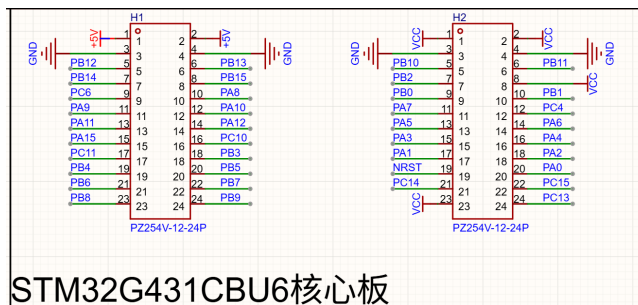
图 3-2: 核心板电路
