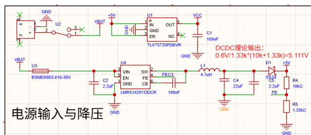
图 3-6: 电源电路
