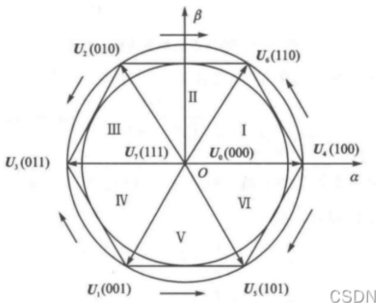
图 2-2: SVPWM 基本矢量和扇区划分图
