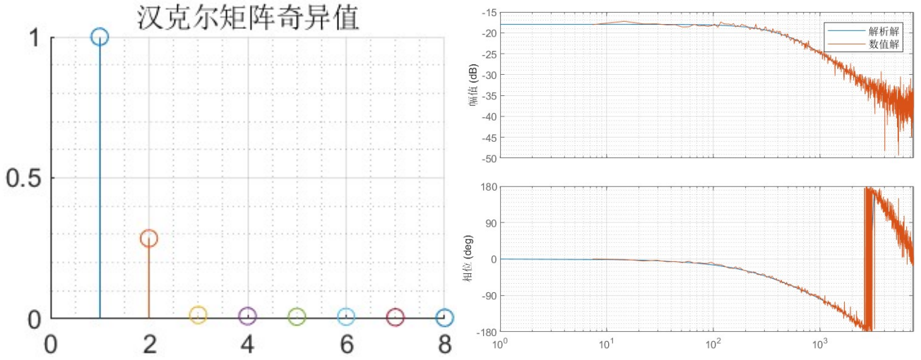
图 4-19: Q 轴工作点 0V 归一化奇异值分解图（仿真，非理想状态）
