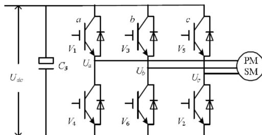
图 2-1: 三相全桥逆变电路
