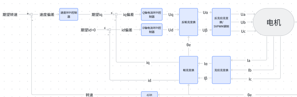
图 3-1: 经典 FOC 控制结构框图
