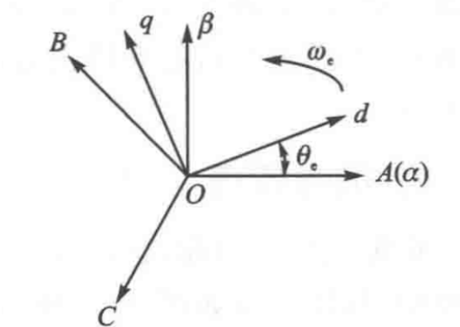
图 1-4: 帕克变换
