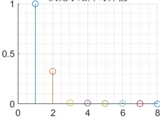
图 4-13: D 轴工作点 0V 归一化奇异值分解图（仿真，非理想状态）
