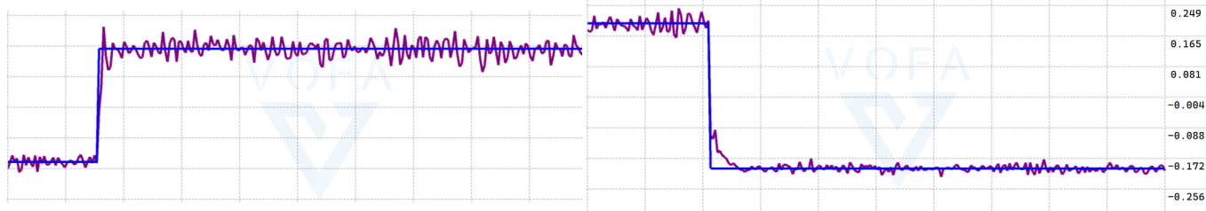
图 3-12: I_d=0.2A 阶跃响应图
