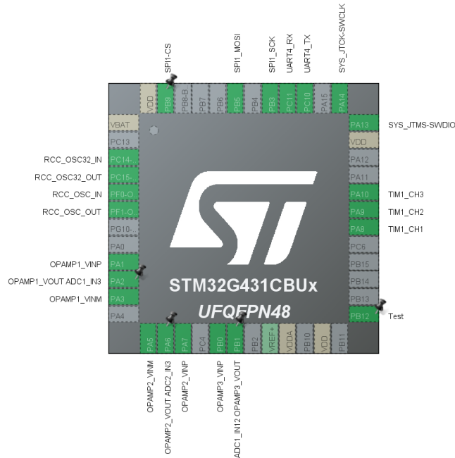
图 3-8: 外设配置图
