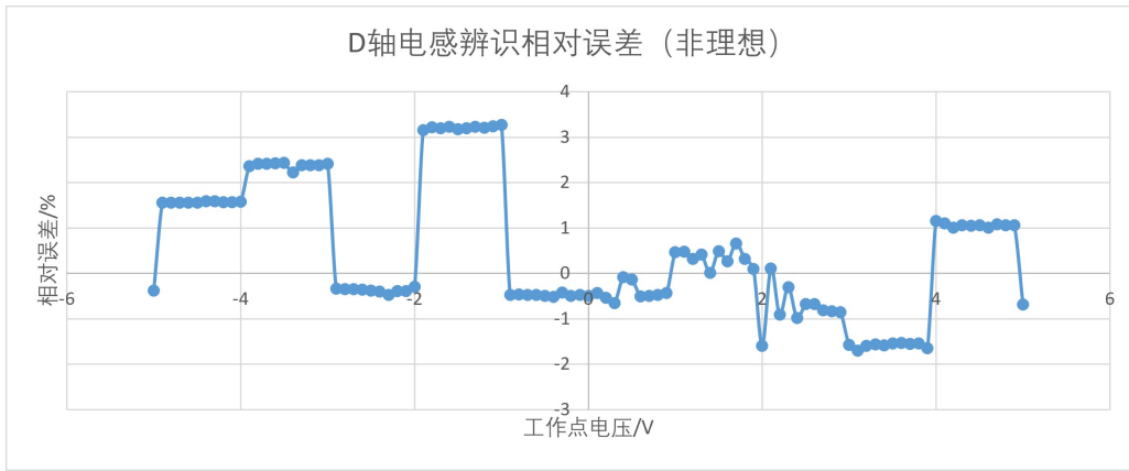
图 4-15: D 轴工作点相对误差分析（仿真，非理想状态）
