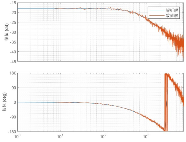
图 4-14: D 轴工作点 0V 解析解与数值解频域对比图（仿真，非理想状态）
