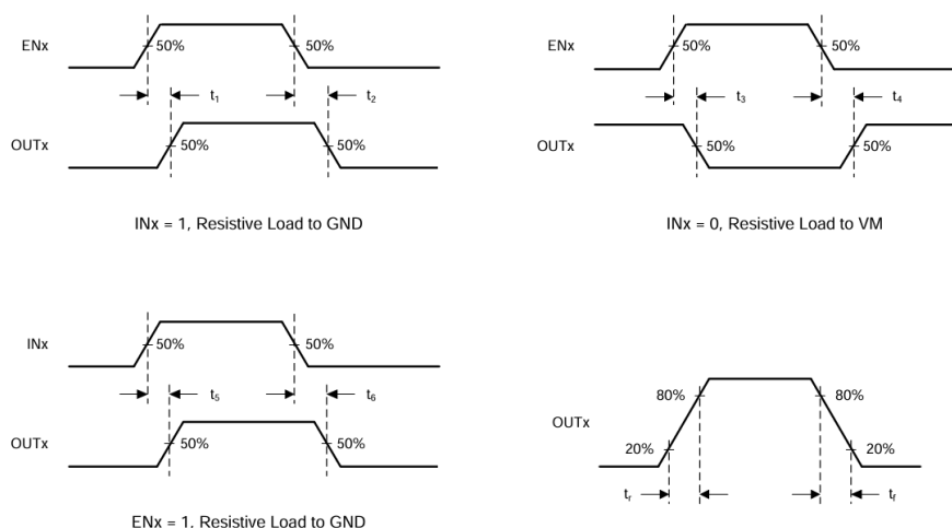
图 4-7: DRV8313 动态特性
