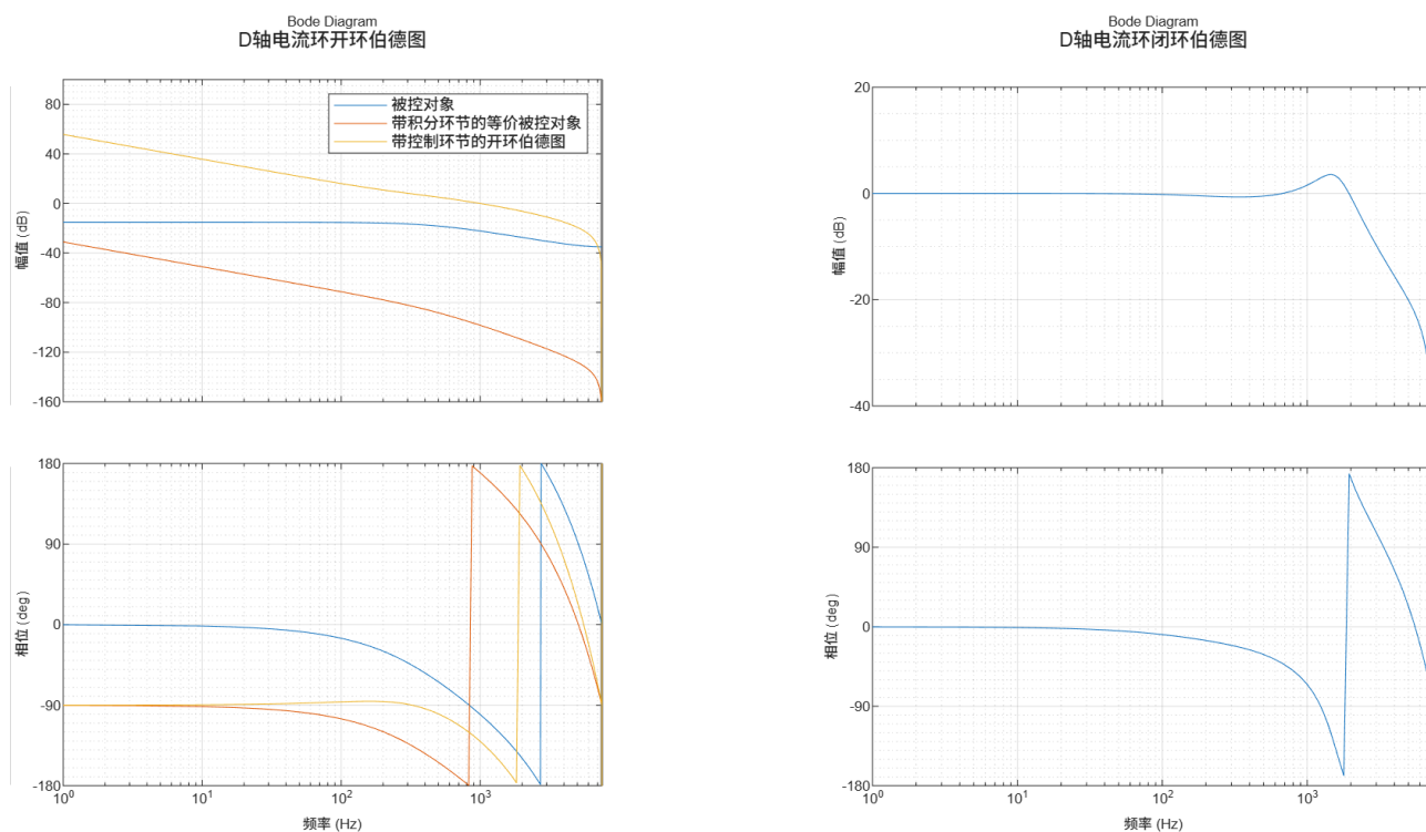
图 5-2: D 轴开-闭环频率特性
