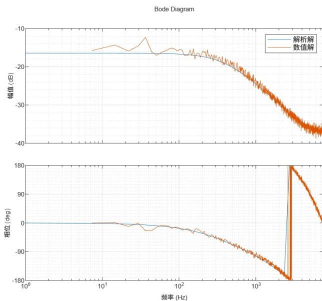
图 4-50: Q 轴工作点 2V 数值解和解析解对比
