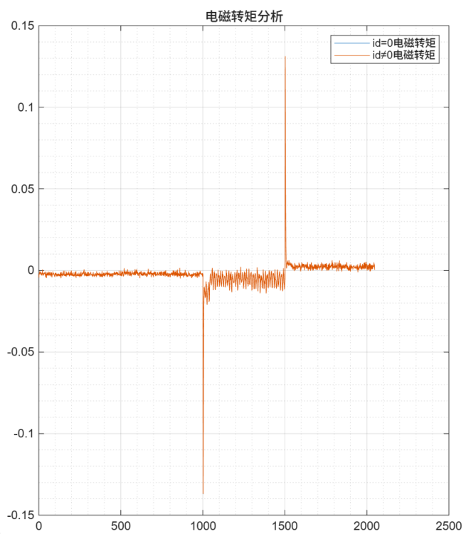
图 5-37: 速度环负向方波电磁转矩对比
