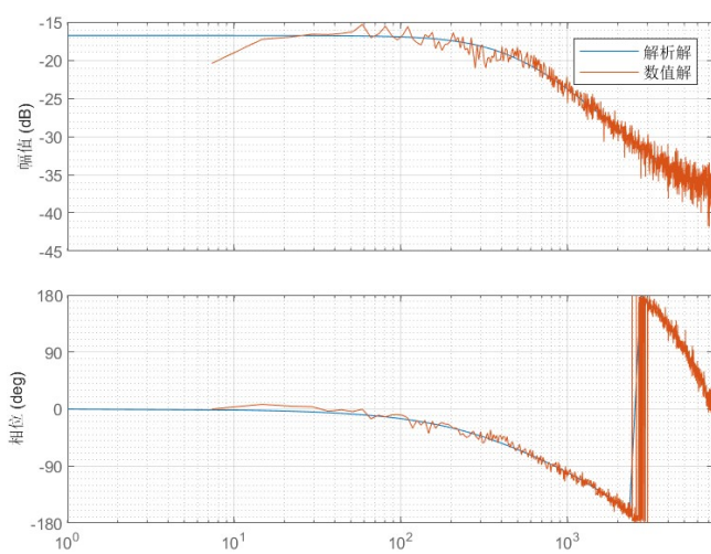
图 4-45: 机械堵转数值解与解析解对比
