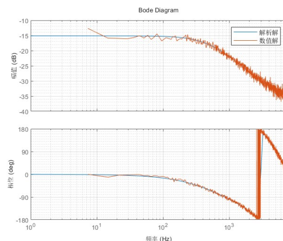
图 4-29: D 轴工作点 2V 数值解和解析解对比
