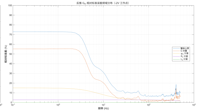
图 5-29: 相对标准误差频域分布曲线 (-2V)
