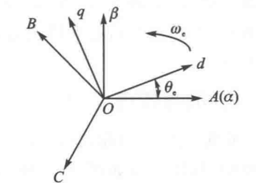
图 1-4: 帕克变换
