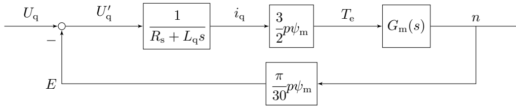
图 5-11: i_d = 0 假设下的 Q 轴电流-速度系统框图
