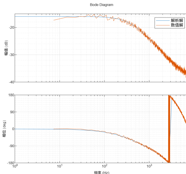
图 4-48: Q 轴工作点 0V 数值解和解析解对比
