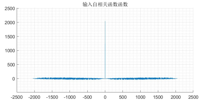
图 4-23: D 轴工作点 0V 输入自相关函数
