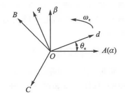
图 1-4: 帕克变换
