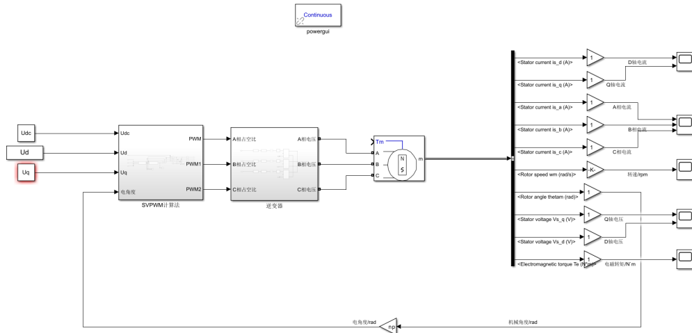
图 4-6: 仿真模型
