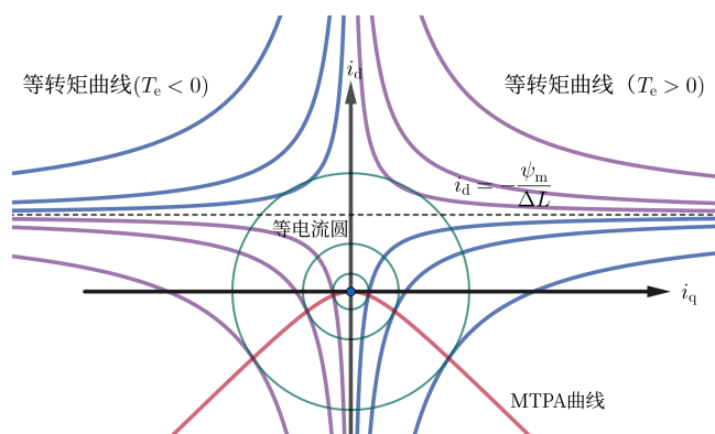
图 6-2: MTPA 几何关系
