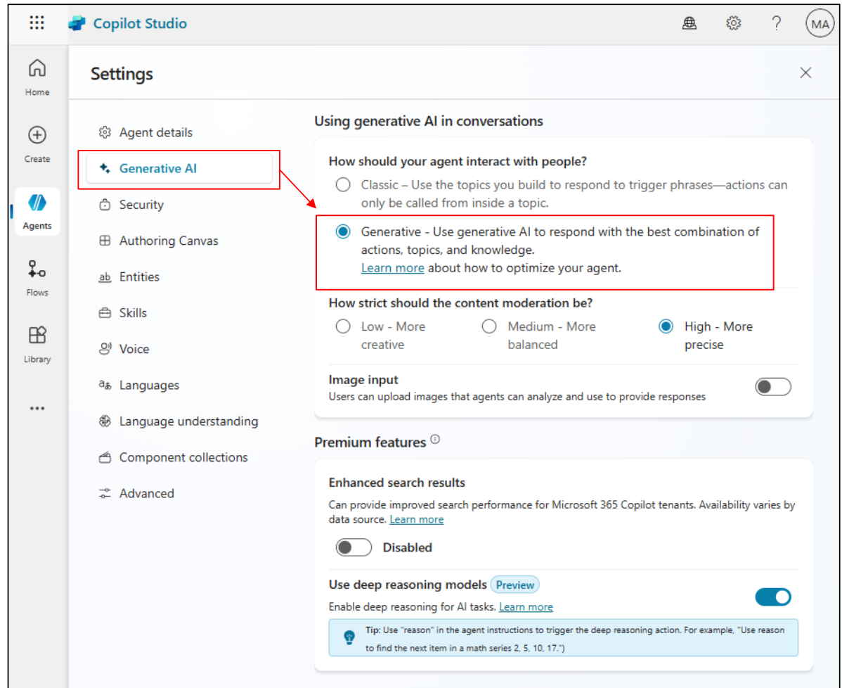
[Agent 설정] – [Generative AI] 에서 Classic에서 Generative로 변경
