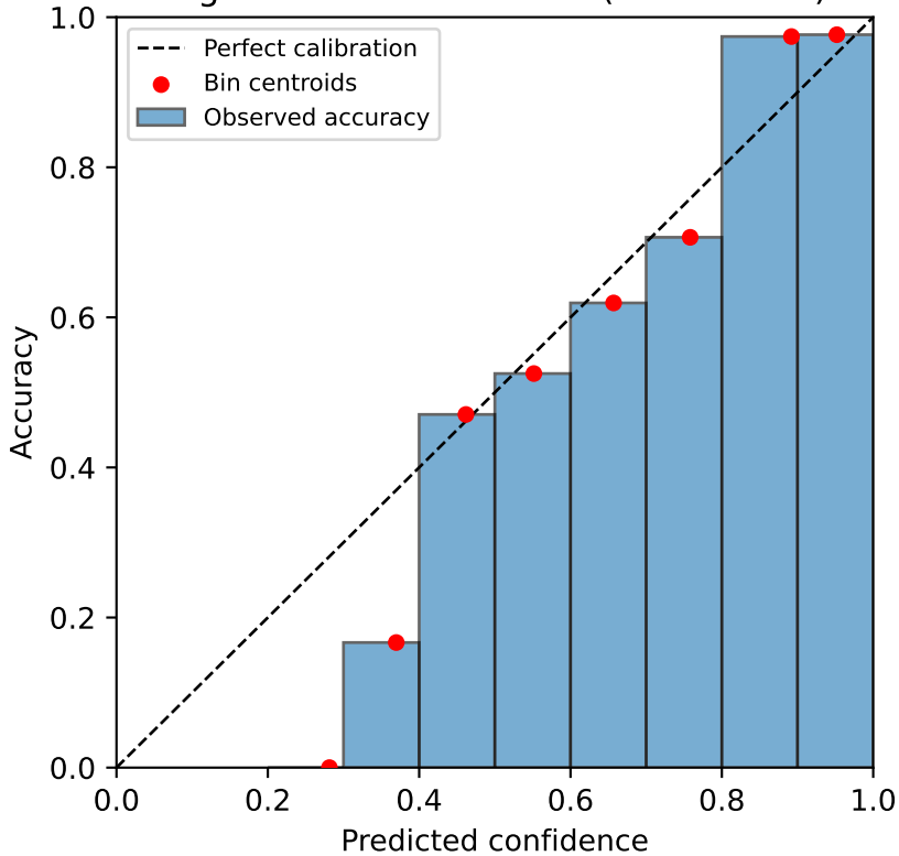
organamnist — baseline (ECE=0.055)
