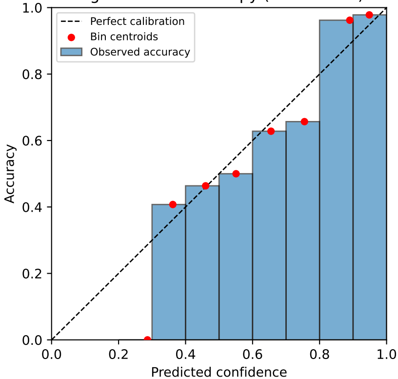
organamnist — entropy (ECE=0.046)
