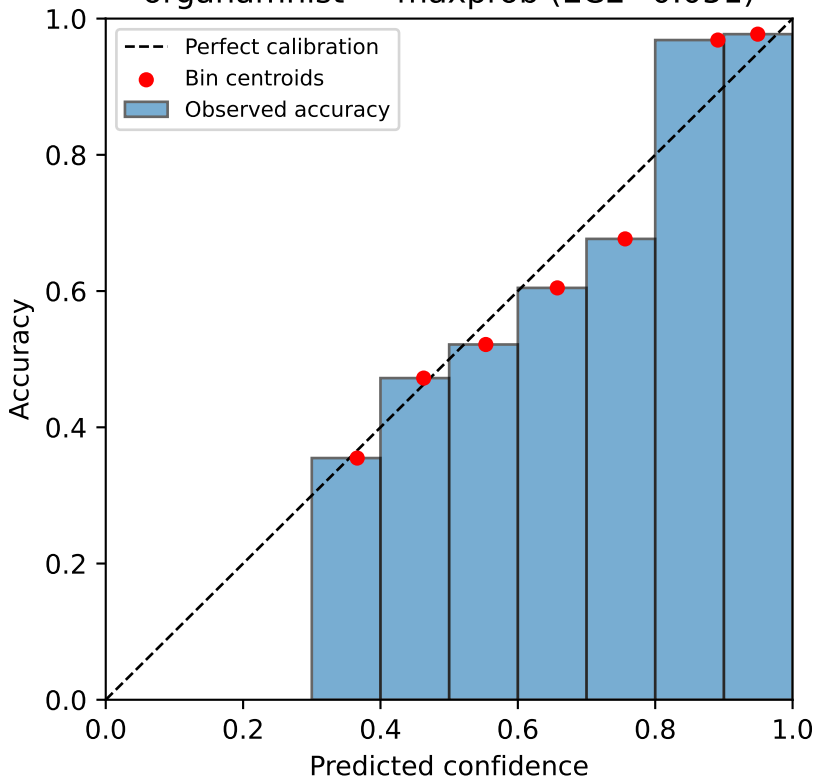
organamnist — maxprob (ECE=0.051)
