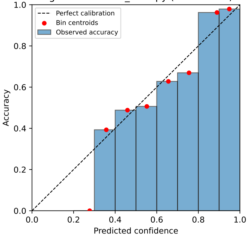
organamnist — ts_entropy (ECE=0.046)
