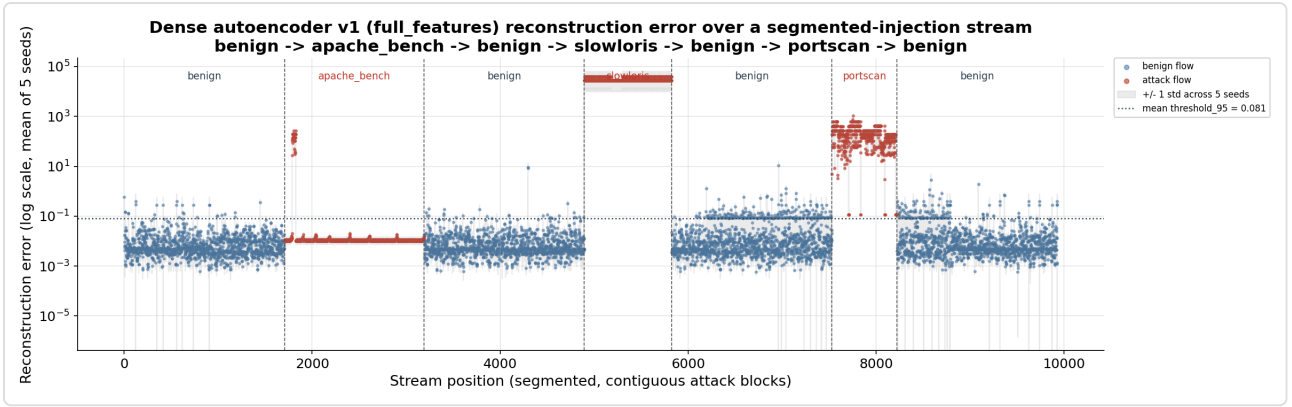
Şekil 3.2 — Aynı segmented akış, Dense autoencoder v1 ile değerlendirilmiş. apache_bench bloğu neredeyse tamamen düz ve deterministik bir çizgi oluşturuyor (5 seed üzerinden recall standart sapması = 0.0000) — VAE'nin daha gürültülü bulutunun aksine (reparameterization'ın stokastik örneklemesinden kaynaklanıyor) — ama hata seviyesi benzer şekilde eşğin çok altında kalıyor.
