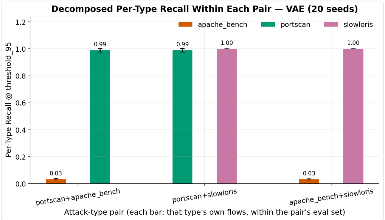
Şekil 2.2 — Aynı ikililerin recall'ü, çift içindeki her tip için ayrı ayrı (decomposed) gösteriliyor. apache_bench'in kendi recall'ü ~%3.2'de sabit kalıyor — poolanmış grafikteki "iyileşme" burada kayboluyor.
