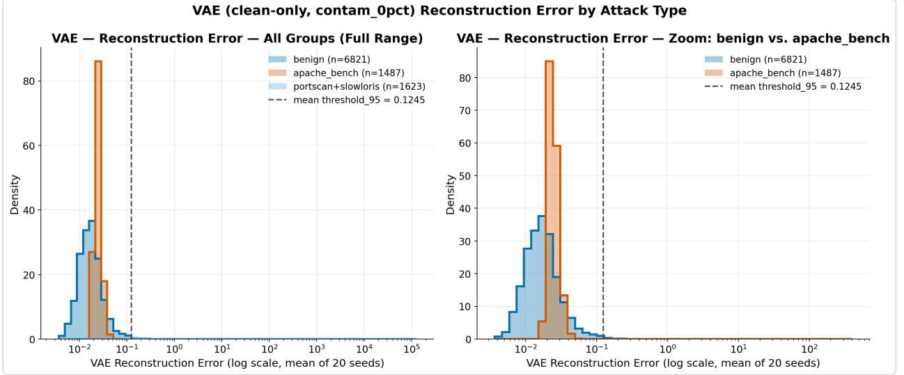
Şekil 4.2 — VAE reconstruction error dağılımı (log ölçek, 20 seed ortalaması), benign / apache_bench / portscan+slowloris (birleşik) için. apache_bench, benign dağılımıyla neredeyse tamamen örtüşüyor.
