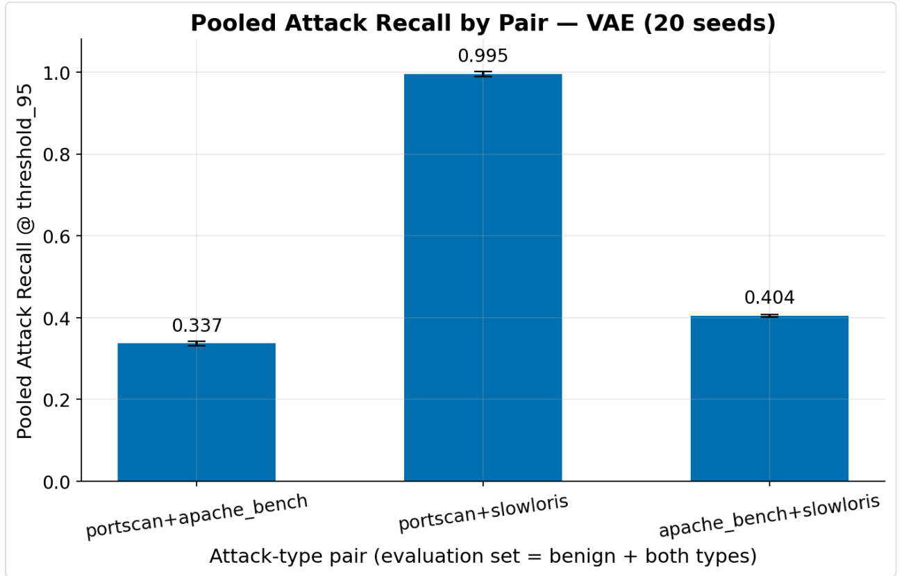
Şekil 2.1 — VAE, 3 ikili kombinasyon için poolanmış (pooled) recall. apache_bench içeren ikililerde recall %34-40 gibi görünüyor.
