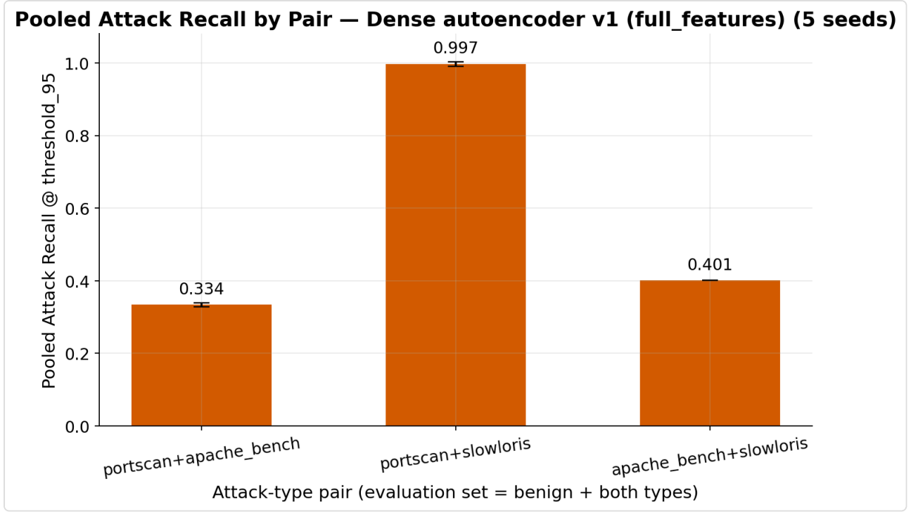
Şekil 2.3 — Dense v1 için poolanmış recall, VAE ile aynı örüntü.
