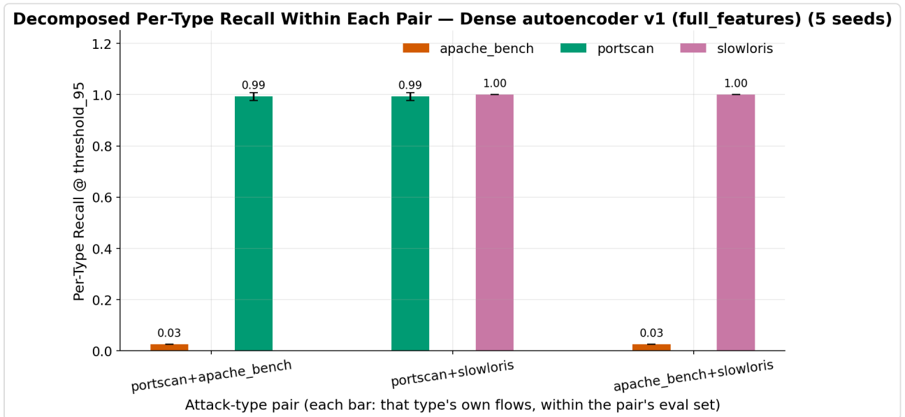
Şekil 2.4 — Dense v1 için ayrıştırılmış recall; apache_bench yine sabit düşük kalıyor.
