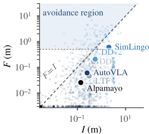
(d) all cells on the two axes
