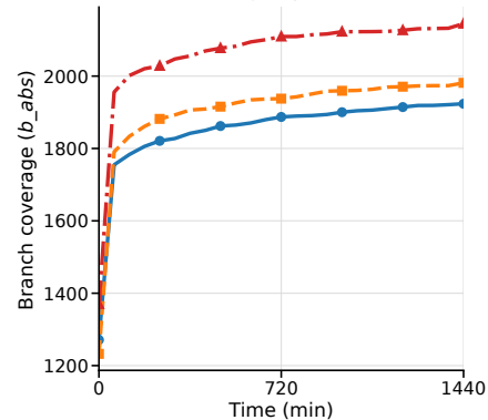
Lighttpd1
