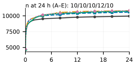
(g) Kmailio
