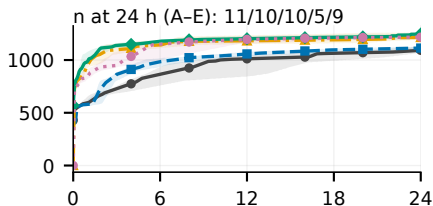
(g) Kmailio
