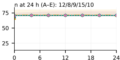
(d) Pure-FTPd
