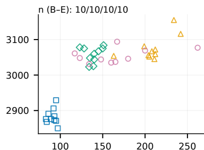
(i) Lighttpd1
