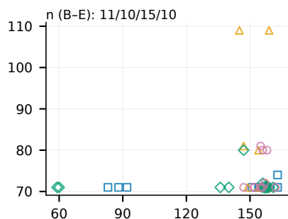
(d) Pure-FTPD
