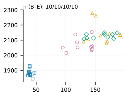
(i) Lighttpd1
