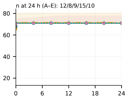
(d) Pure-FTPd
