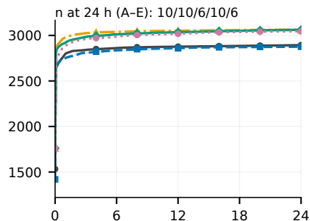
(i) Lighttpd1
