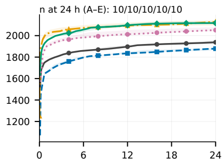
(i) Lighttpd1
