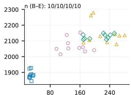
(i) Lighttpd1
