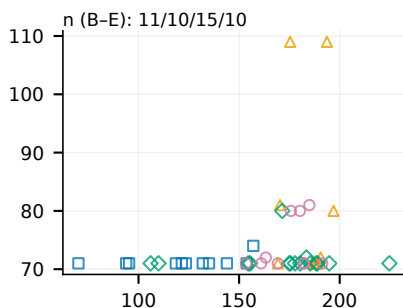
(d) Pure-FTPd
