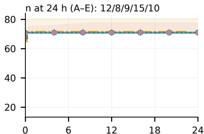
(d) Pure-FTPd
