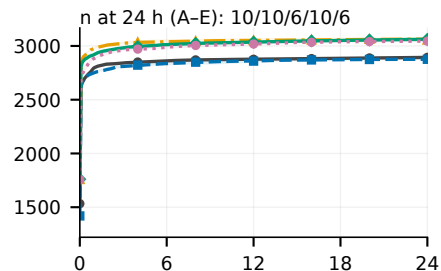
(i) Lighttpd1
