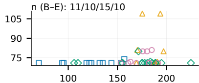
(d) Pure-FTPD
