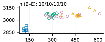
(i) Lighttpd1
