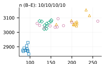
(i) Lighttpd1
