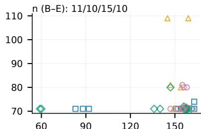
(d) Pure-FTPD
