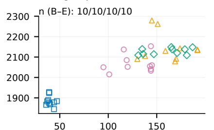
(i) Lighttpd1
