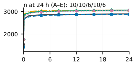
(i) Lighttpd1
