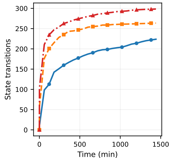
Pure-FTPd
