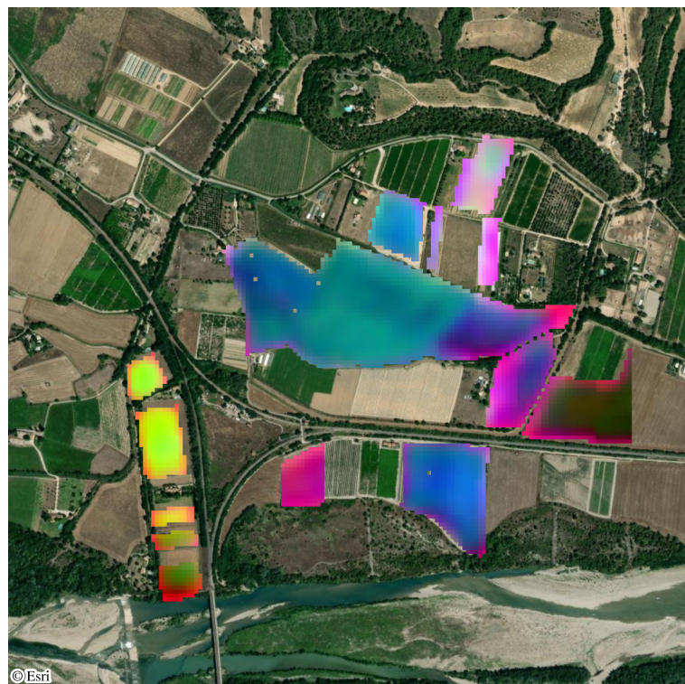
Embedding PCA
