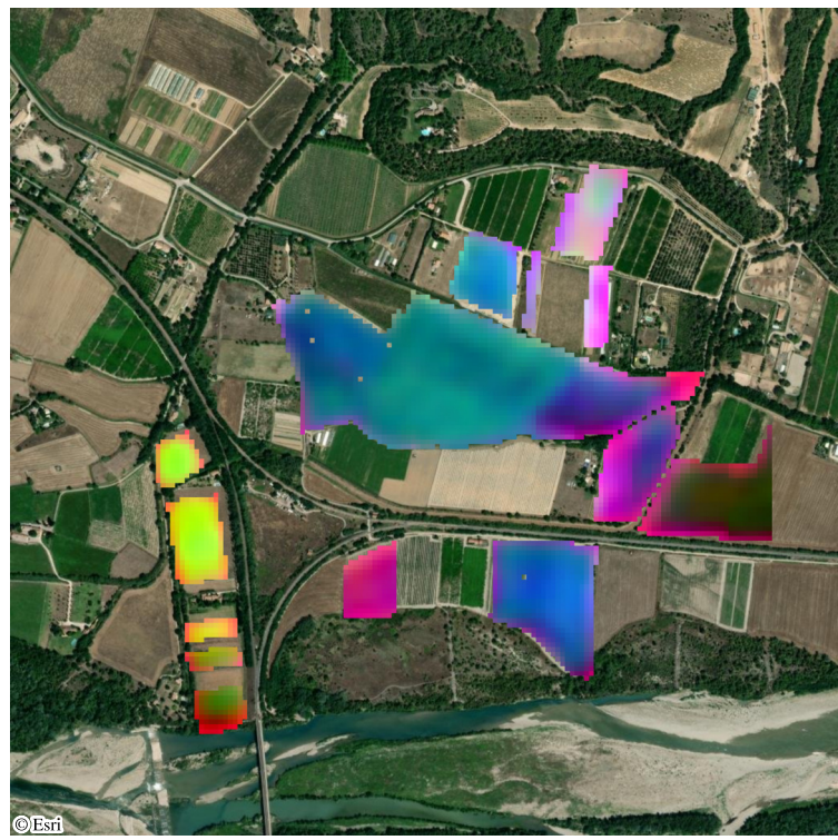
Embedding PCA
