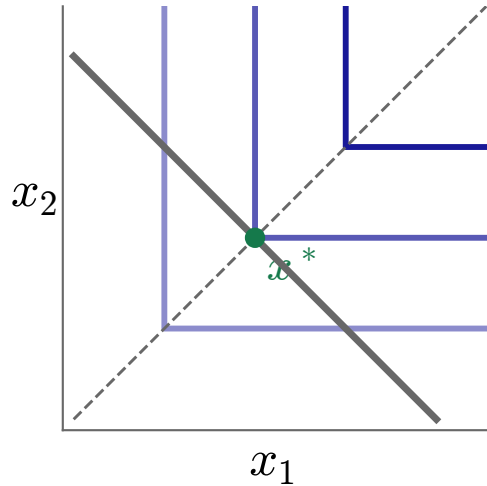
Leontief kink
