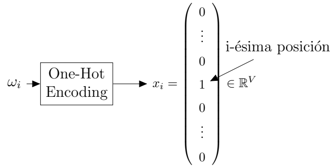
Figura 5.1: Ejemplo de codificación one-hot asociado a una palabra.
