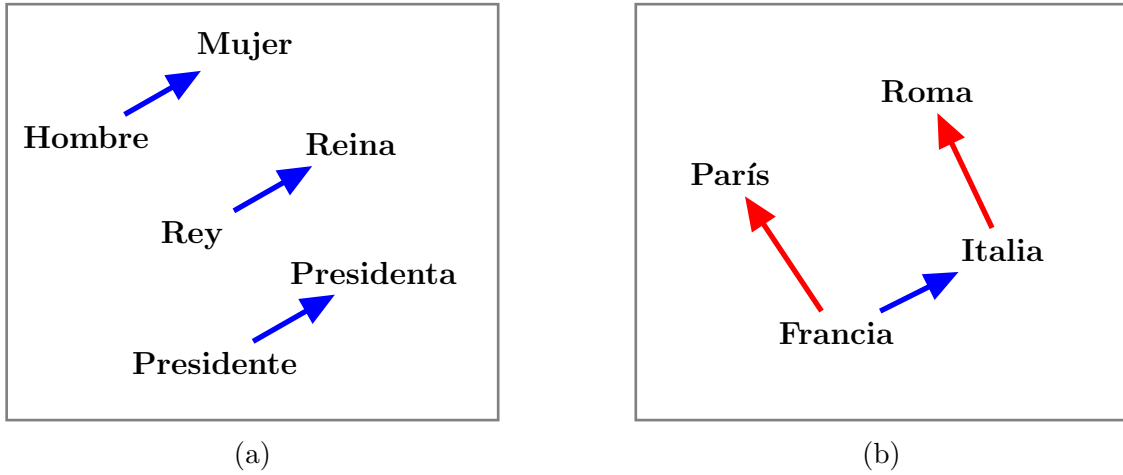
Figura 5.2: Ejemplo de interpretación geométrica basada en semántica. (a) Relaciones de género; y (b) analogías.
