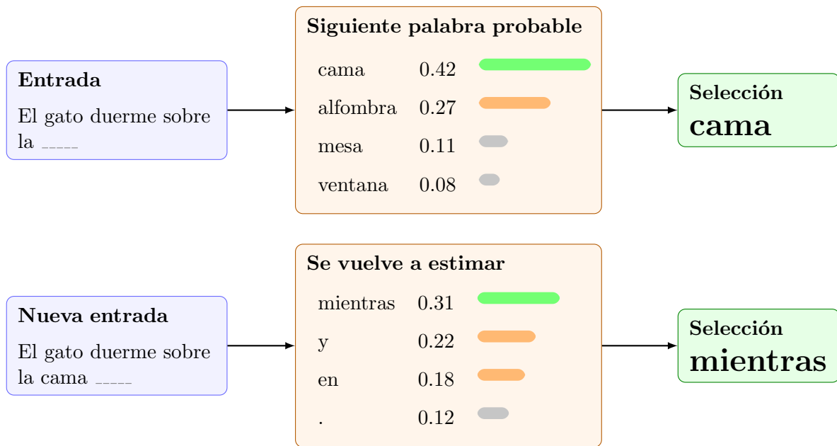
Figura 5.6: Ejemplo de procedimiento autorregresivo de un modelo de lenguaje.
