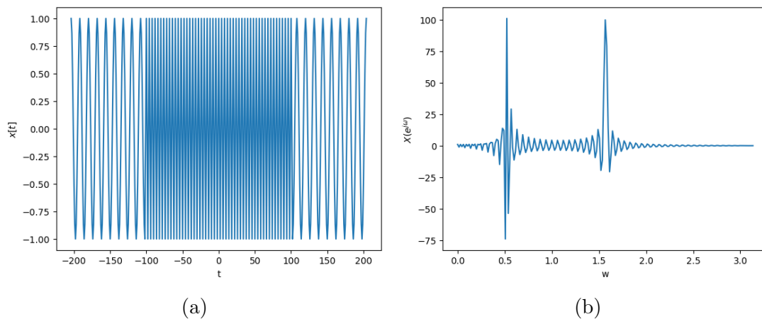
Figura 5.2: Señal no estacionaria. (a) Comportamiento temporal, y (b) Transformada de Fourier.
