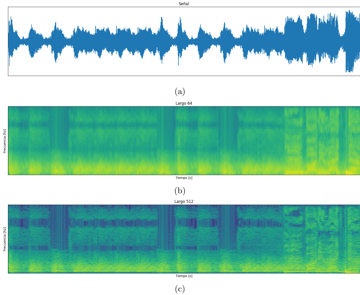
Figura 5.3: Ejemplo de espectrograma. (a) Señal temporal, (b) espectrograma para una ventana de largo 64, y (c) espectrograma para una ventana de largo 512.
