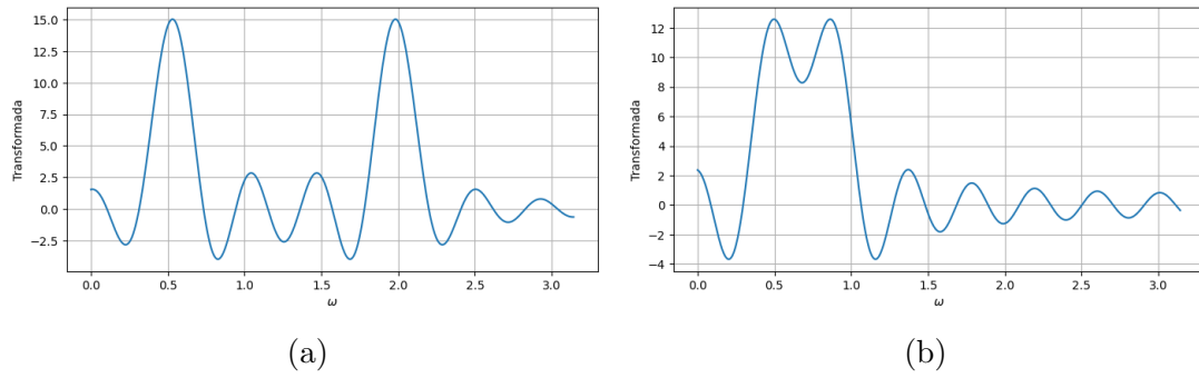
Figura 5.1: Transformada de Fourier (en valor absoluto) de suma de dos sinusoides ventaneada. (a) Con las sinusoides lejos, y (b) con las sinusoides cerca.
