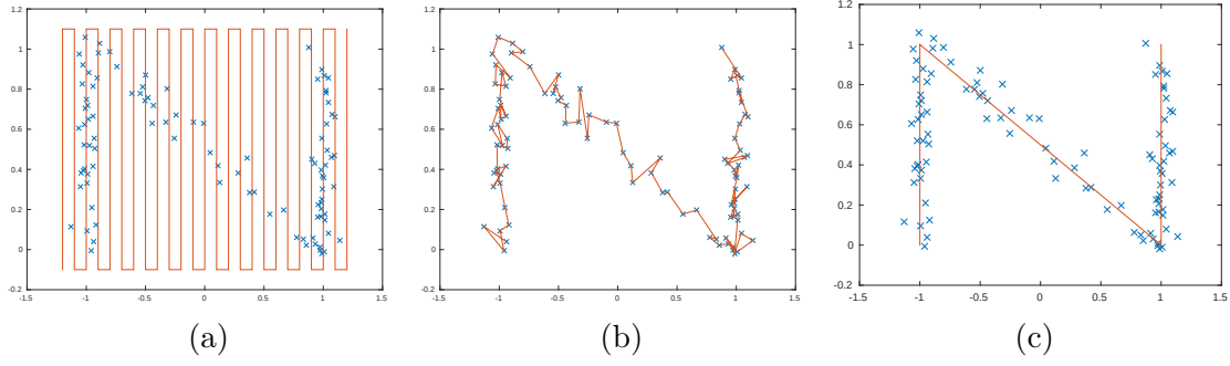
Figura 4.3: Ejemplo de aprendizaje en una tarea de reducción de dimensión [30]. (a) Para un algoritmo con overfitting ; (b) para uno con encoder biyectivo; y (c) para un algoritmo con correcto manifold learning .
