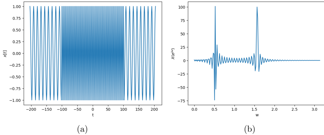
Figura 5.2: Señal no estacionaria. (a) Comportamiento temporal, y (b) Transformada de Fourier.
