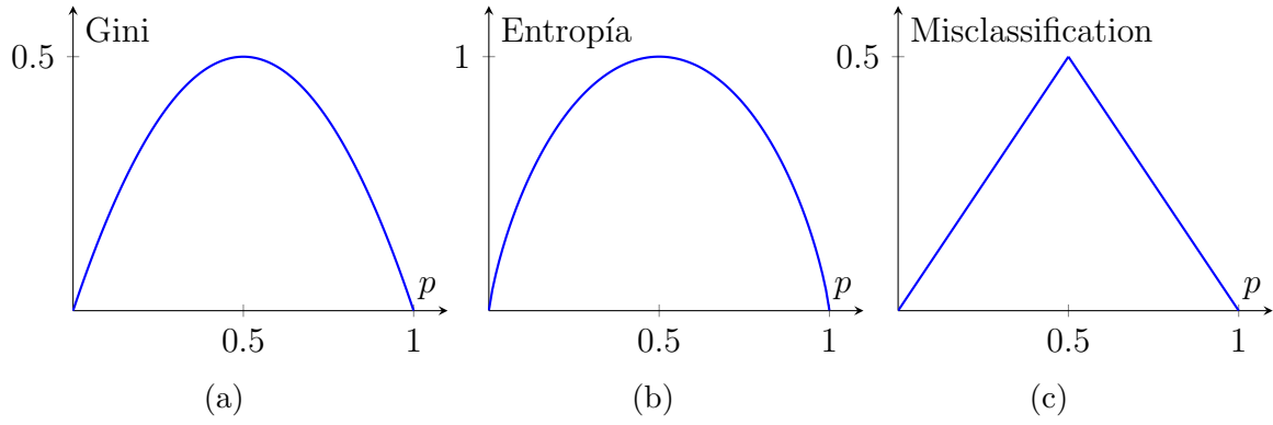
Figura 3.13: Funciones impureza para un problema de clasificación binaria. (a) Impureza de Gini; (b) Entropía; y (c) Misclassification.
