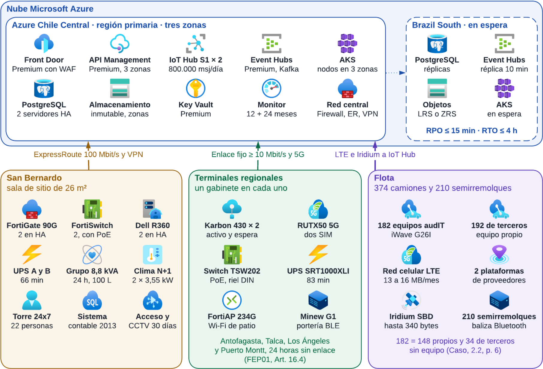
Figura 4.8 Vista general de la arquitectura física: nube primaria y secundaria, San Bernardo, terminales regionales y flota, con los enlaces y su capacidad Fuente: Elaboración propia.
