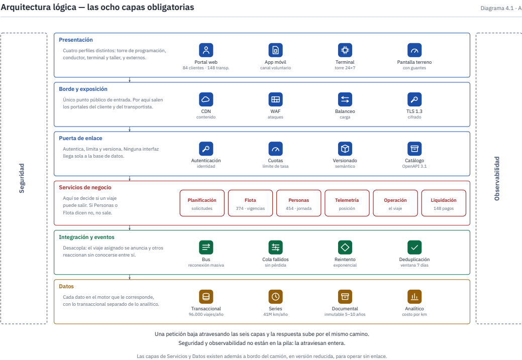
Figura 4.1 Las ocho capas obligatorias del numeral 2.1 transversal, con sus componentes e interfaces, conforme a RT-02.01 Fuente: Elaboración propia.
