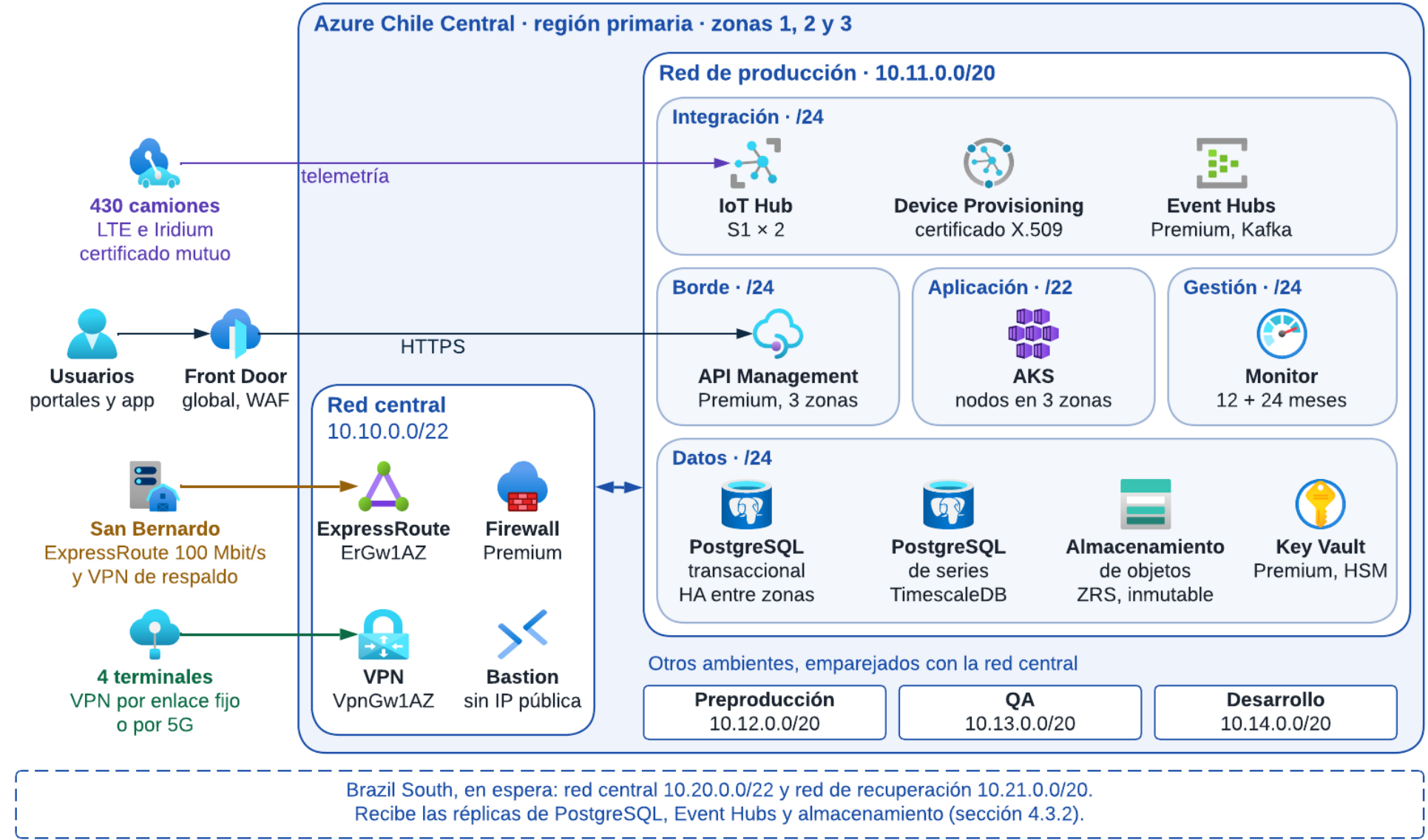
Figura 4.11 Región primaria Azure Chile Central: red central, red de producción, subredes, servicios con su nivel y conexiones con San Bernardo y los terminales Fuente: Elaboración propia.
