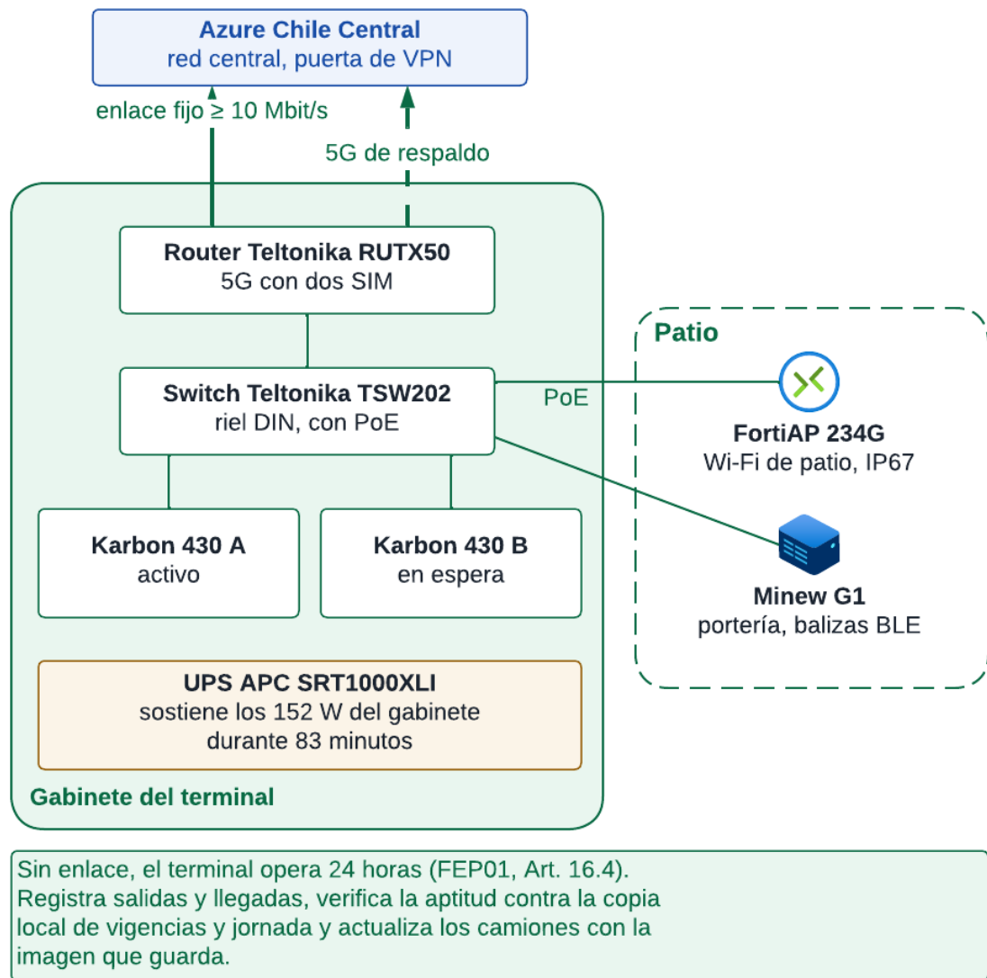
Figura 4.14 Gabinete de un terminal regional, con sus enlaces, el punto de acceso de patio y el lector de portería
