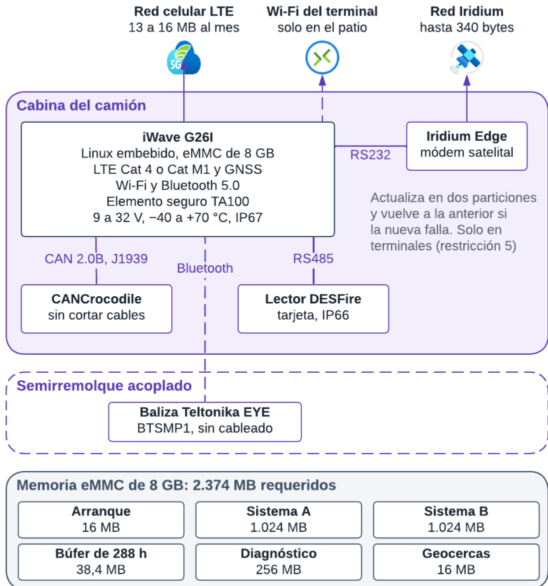
Figura 4.9 Equipo a bordo: iWave G26I, periféricos, interfaces y particiones de la memoria Fuente: Elaboración propia.
