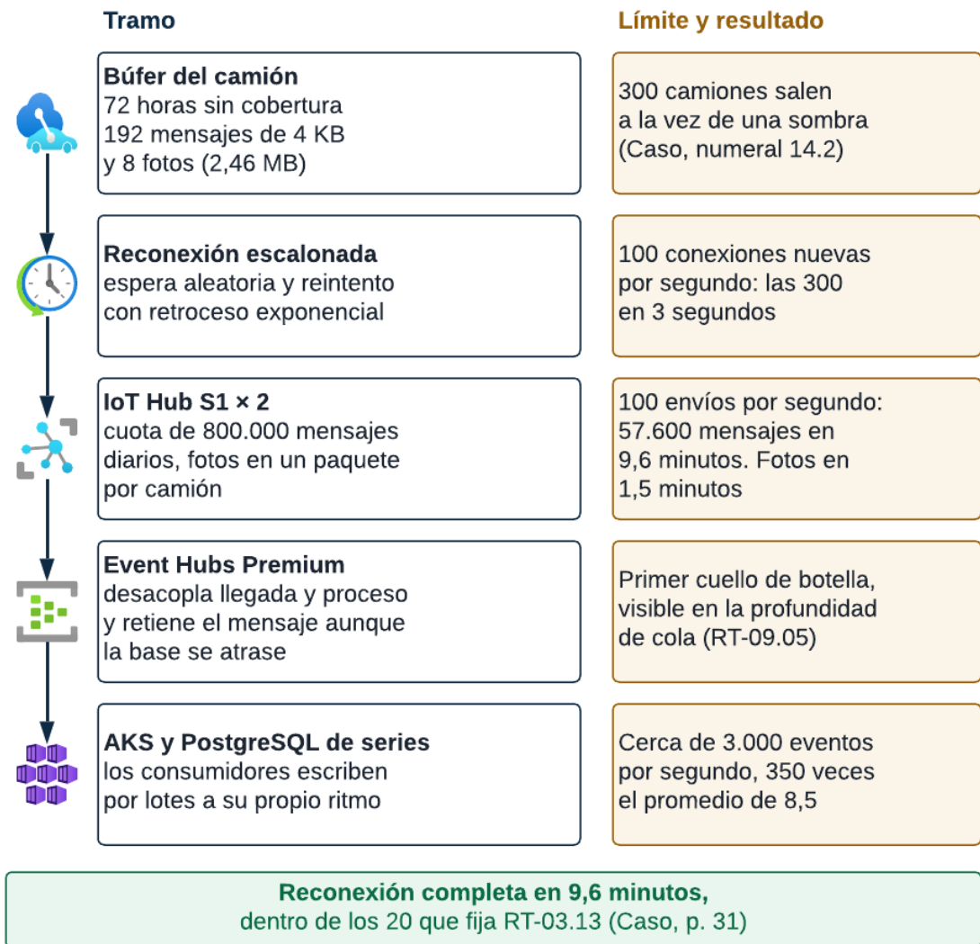
Figura 4.12 Reconexión masiva: del búfer del camión a la base de datos, con los límites de cada tramo
