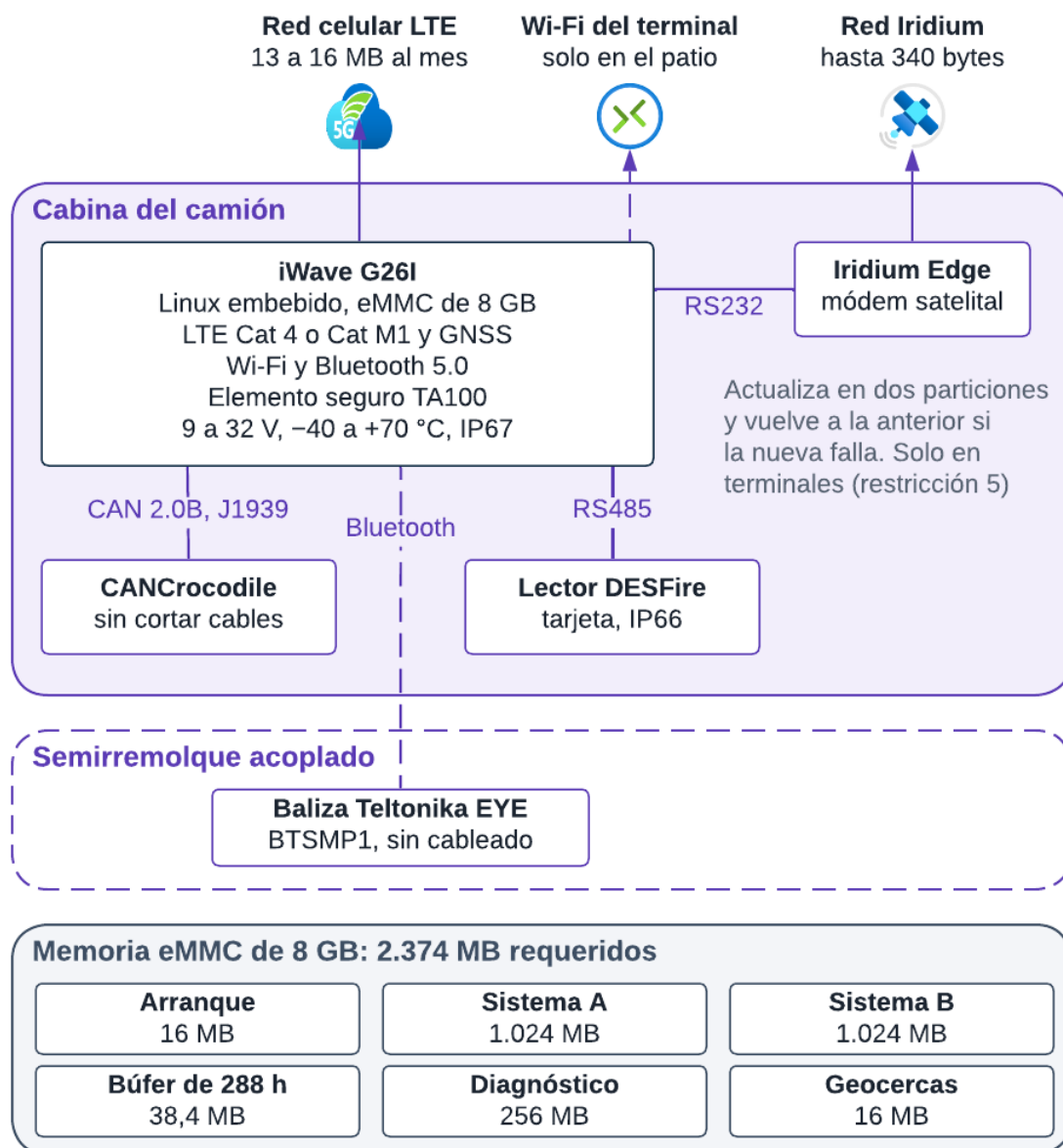
Figura 4.9 Equipo a bordo: iWave G26I, periféricos, interfaces y particiones de la memoria Fuente: Elaboración propia.
