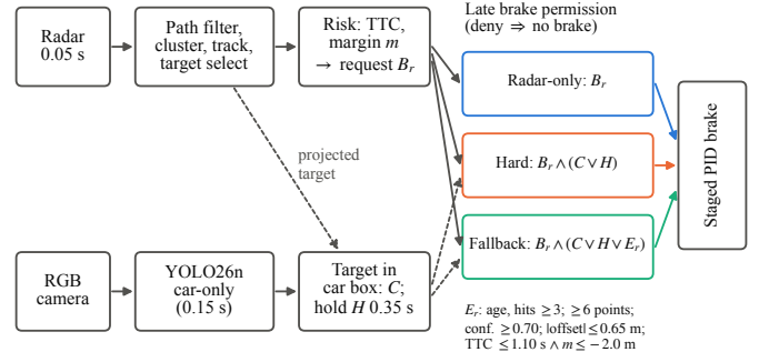
Fig. 1. Chuỗi xử lý dùng chung từ cảm biến đến phanh. Ba chính sách nhận cùng yêu cầu phanh radar B_r và cùng xác nhận car C /giữ H , chỉ khác ở bước cấp quyền cuối: gate cứng từ chối B_r nếu không có box car tại mục tiêu chiếu; fallback còn cấp quyền khi điều kiện khẩn cấp E_r thỏa. Hình giữ nhãn tiếng Anh để đối chiếu với bản nộp.
